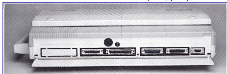
Conexiones, de izquierda a derecha: unidad de expansión (2 conectores), fuente de alimentación monitor PC 1640, fuente propia, salida serie, paralelo y video RGB.
