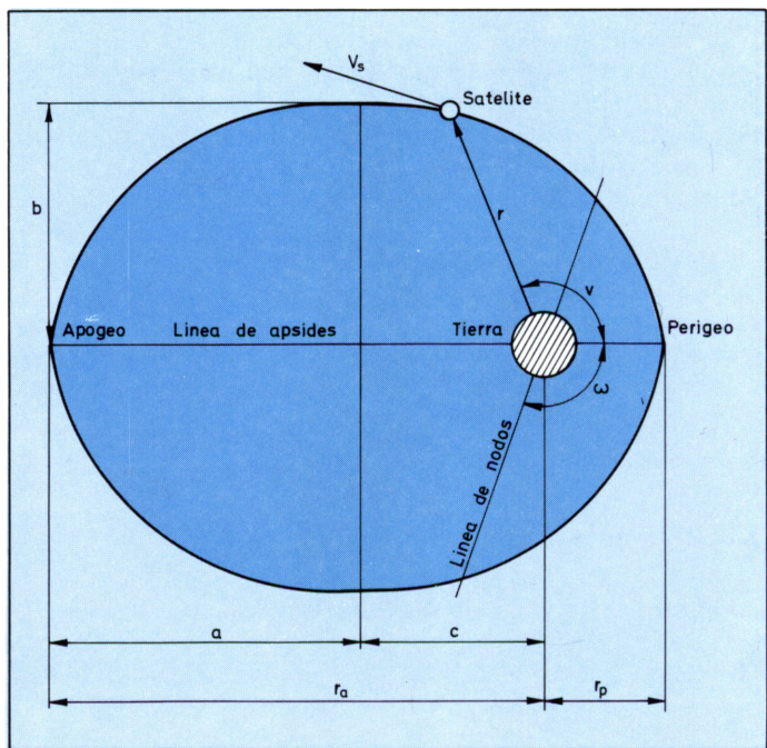
Figura 3. Representación esquemática de la órbita elíptica de todo satélite lanzado desde la Tierra. En el dibujo se indican los puntos más notables de la misma como son: el perigeo, el apogeo, las líneas de nodos y el radio vector ( r ).
