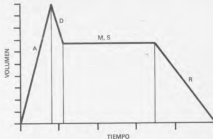
Figura 7.—Cuatro fases que describen la envolvente de un sonido: ataque, decaimiento, mantenimiento o sostenimiento y relajación.
