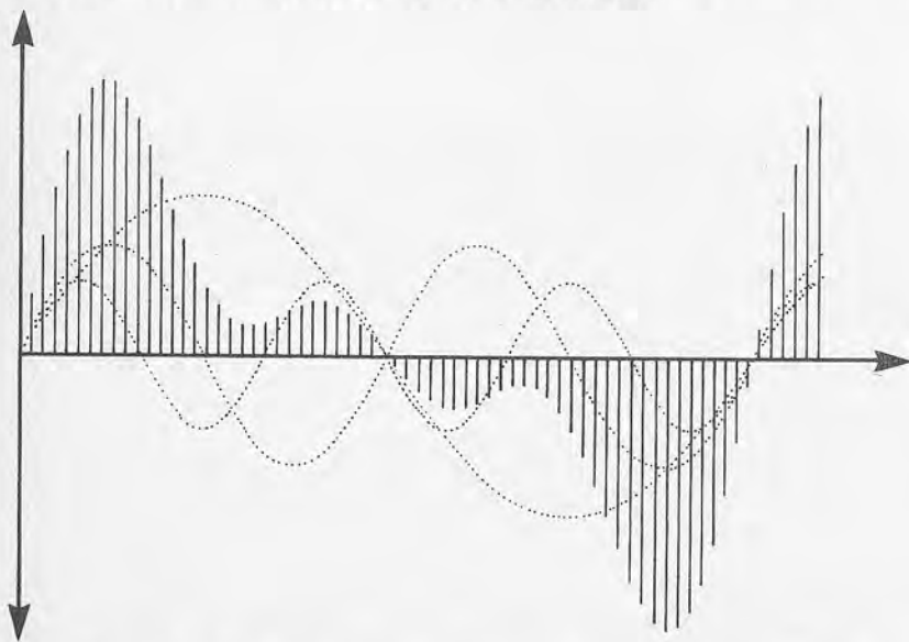
Figura 9.—Otro ejemplo de síntesis aditiva. Hemos puesto los tres primeros armónicos con pesos respectivos 1, 3/4 y 1/2 (la amplitud máxima del tercer armónico es, por tanto, la mitad de la del fundamental). Tanto aquí como en la figura 8 los armónicos están en fase (parten de cero en igual dirección a la vez en el mismo instante). Con ondas desfasadas se obtiene una onda resultante distinta (y un resultado ligeramente distinto para el oído).
