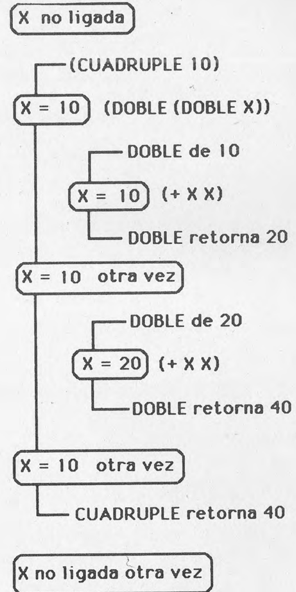
Figura 1.—Ligaduras locales en la función CUADRUPLE.
