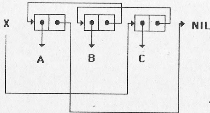
Figura 8.—Comparación de REVERSE y NREVERSE.
