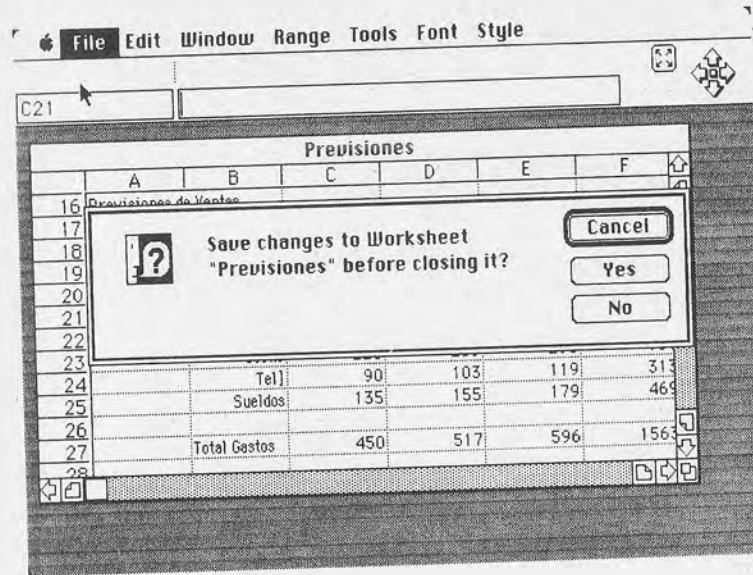
Figura 6.—Marco interactivo
