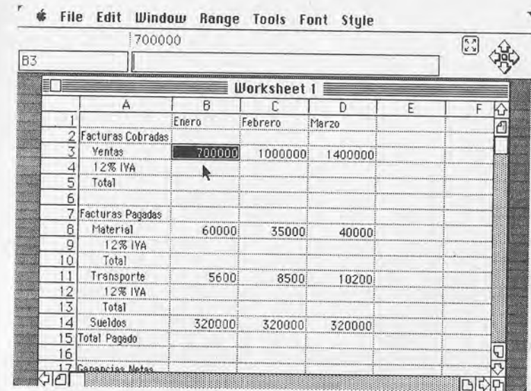
Figura 8.—Datos numéricos
