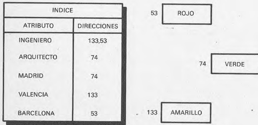
Figura 8.—Estructuras de listas invertidas.
