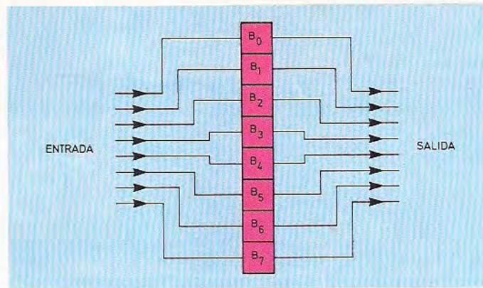
Esquema general de un registro para palabras binarias de ocho bits. Cada uno de los bits, cero o uno se almacena en un elemento biestable.
