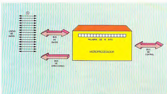
Arquitectura interna típica de un microprocesador de 16 bits. La longitud de las palabras determina el tamaño del bus de datos.
