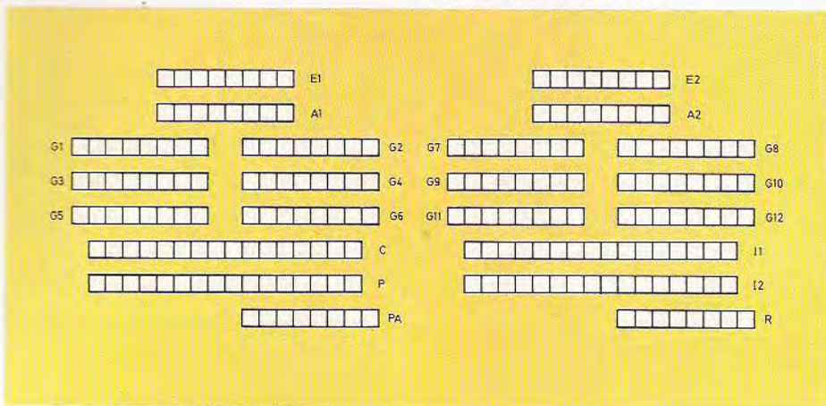
El doble juego de registros internos constituye una de las características básicas del microprocesador Z-80. A los registros generales (G1, ..., G6) se les suele llamar B, C, D, E, H y L.
