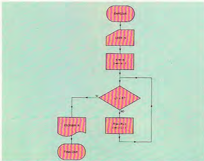
Un algoritmo puede también representarse en forma de diagrama de flujo. El de la figura corresponde al cálculo del factorial de un número N.
