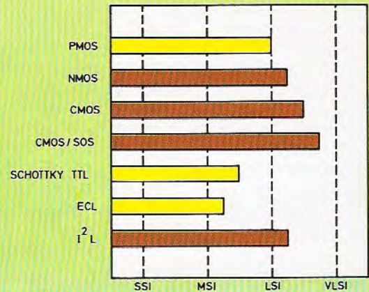
En el eje horizontal se representa el grado de integración comparativo de componentes electrónicos que alcanza cada una de las familias lógicas de las tecnologías bipolar y MOS, habitualmente utilizadas en la fabricación de microprocesadores.
