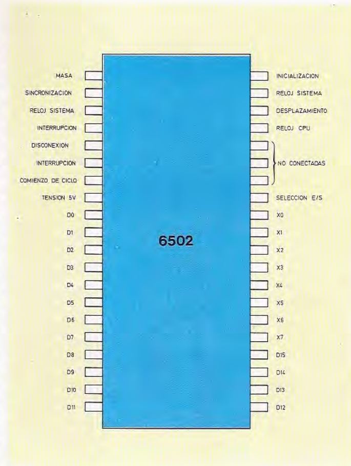
Esquema de las conexiones externas del microprocesador 6502. El bus de direcciones se ha representado con la letra D (D0, D1, ..., D5) y el de datos con la letra X (X0, ..., X7).
