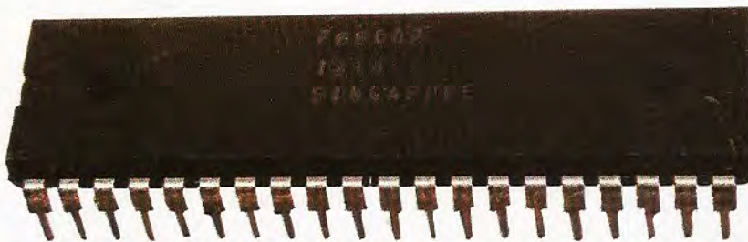
El microprocesador 6800, una vez encapsulado. El aspecto exterior de este microprocesador de 8 bits es similar al de cualquier otro circuito integrado de 40 patillas.
