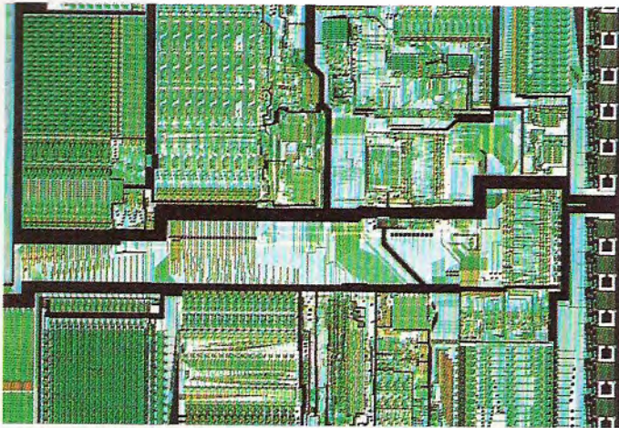
Circuito completo, antes de la fase de encapsulado, de un microprocesador de 16 bits. Su tamaño real es de algunos milímetros cuadrados en los que se alojan varios miles de transistores.
