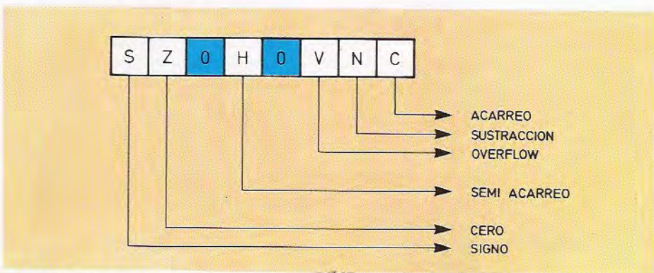
El registro de estado del microprocesador Z-80 consta de 8 bits de los que sólo se utilizan seis.
