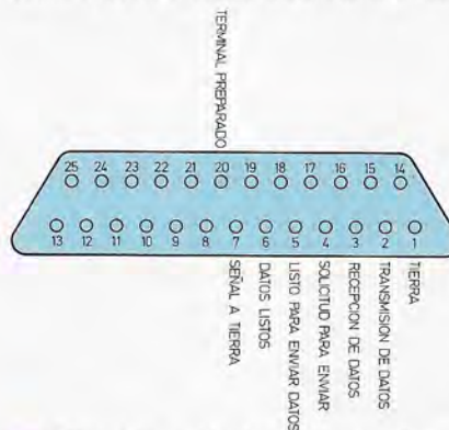
Conector estándar correspondiente a un sistema de comunicación en formato serie según la norma RS/232C. En el gráfico se indica el cometido de los terminales más relevantes.
