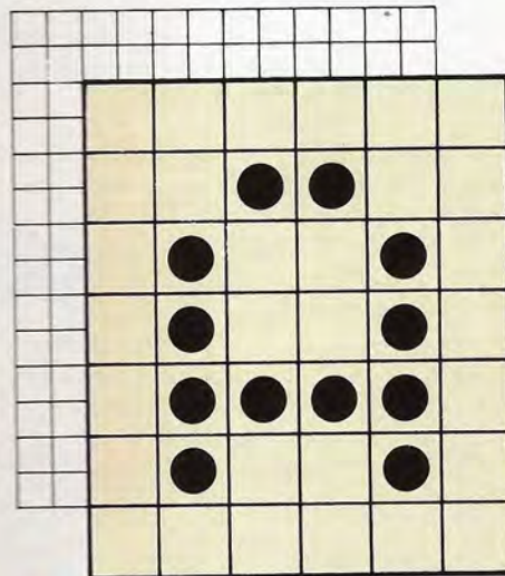
La formación de los caracteres en las impresoras matriciales tiene lugar por medio de una serie de puntos. Estos son estampados sobre el papel con unos minúsculos martillos (las agujas) que presionan a la cinta entintada sobre el papel al ser activados por señales procedentes del ordenador.
