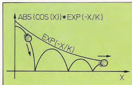
Para que sea posible contemplar la amortiguación de los rebotes de la pelota, habrá que multiplicar la función \text{ABS}(\text{COS}(X)) por la expresión exponencial \text{EXP}(-X/K) .
