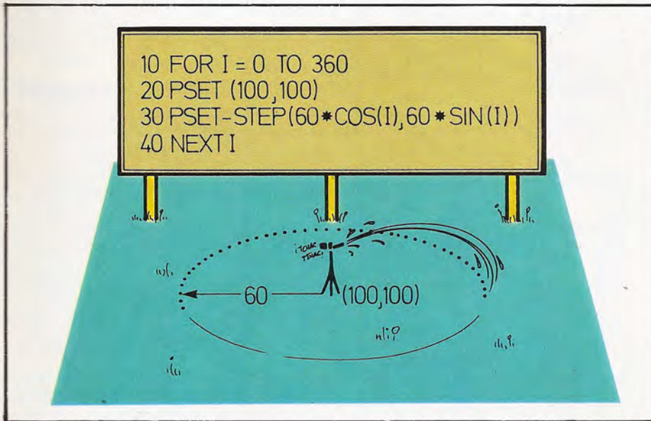
En el texto se explica cómo crear una circunferencia a base de puntos. Los puntos se definen por medio de sus coordenadas relativas al punto central.
