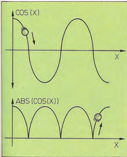
Representación gráfica de las funciones \text{COS}(x) y \text{ABS}(\text{COS}(x)) . Por medio de ellas es posible simular la trayectoria de una pelota botando.
