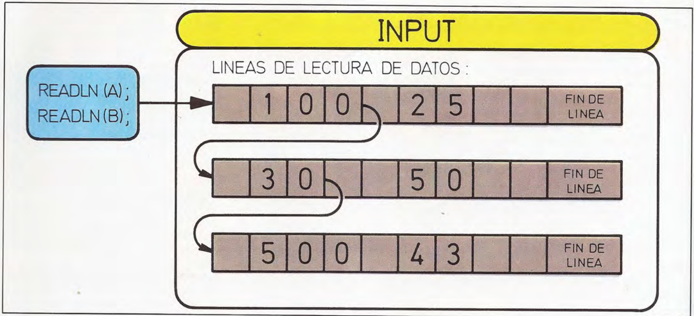
La sentencia READLN permite una lectura selectiva de los datos de entrada, saltando automáticamente a la línea siguiente tras leer el dato ordenado.
