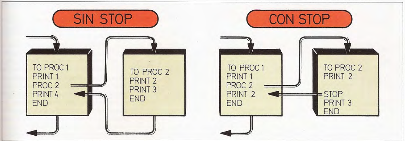
El uso del comando STOP permite abandonar un procedimiento, antes de que éste llegue al final del mismo delimitado por la orden END.
