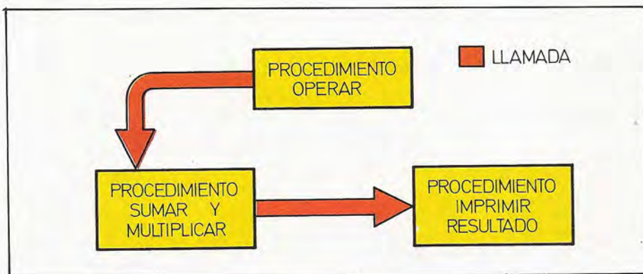
Un procedimiento puede activar a otro distinto y éste, a su vez, a un tercero; y así sucesivamente, creando estructuras más complejas.
