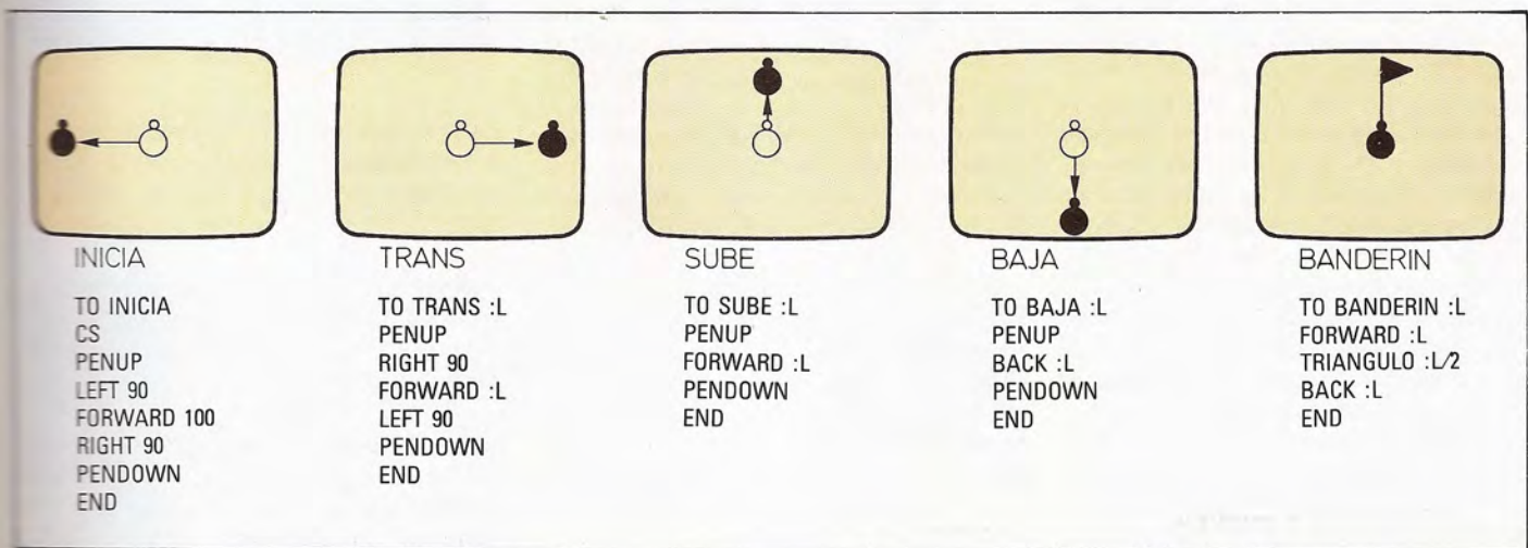
Cinco procedimientos elementales o «de utilidad», adecuados para la creación de superprocedimientos gráficos.
