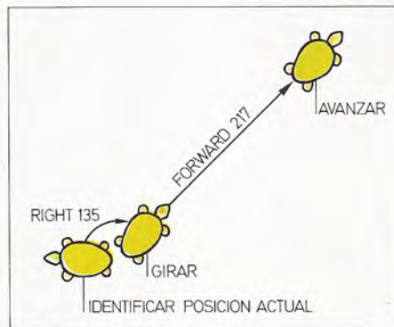
Secuencia de pasos necesarios para situar a la tortuga en un determinado punto de la pantalla.
