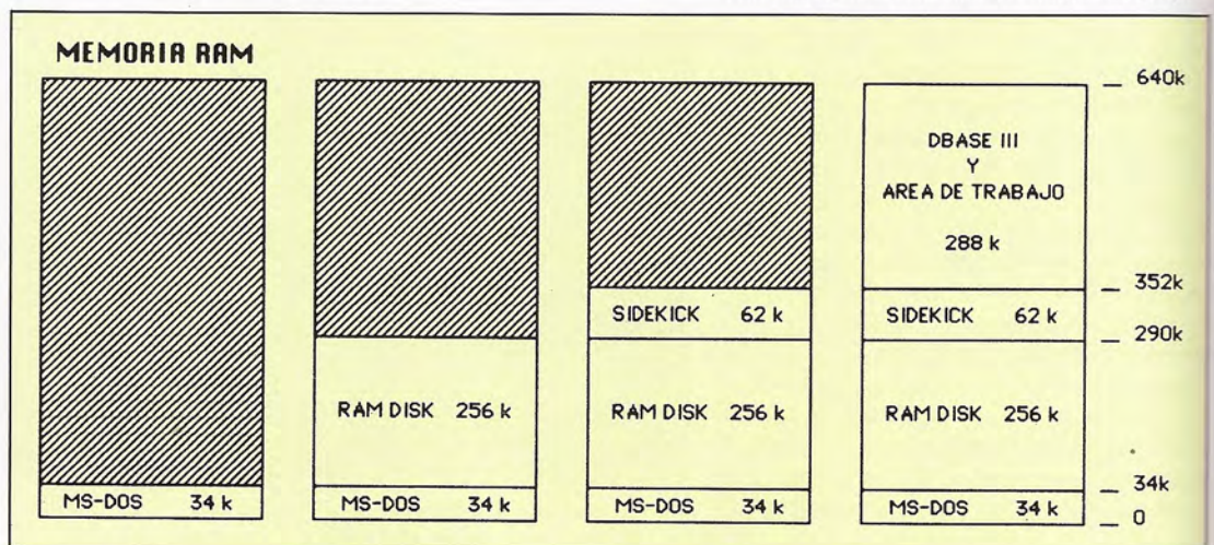
Los paquetes de útiles de escritorio corresidentes en RAM han llegado a convertirse en auxiliares irrenunciables para muchos usuarios.
