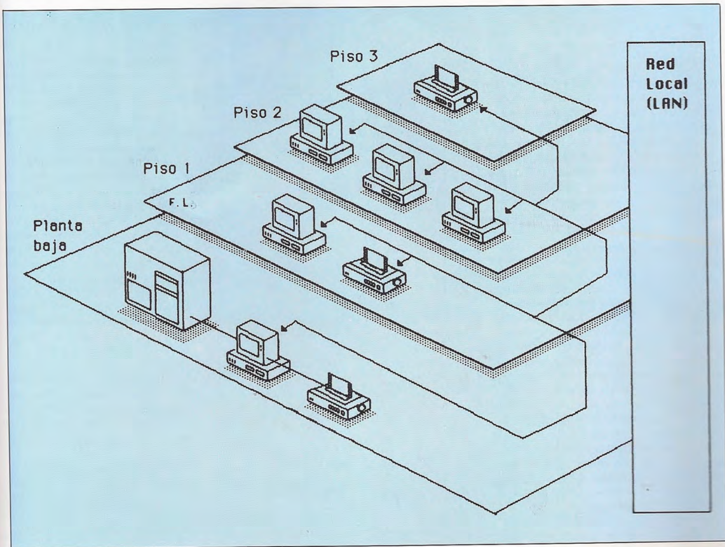
En la figura se esquematiza un ejemplo de red local: en la planta baja se sitúa el «centro de cálculo principal», en la primera planta existe una pantalla con impresora, en la segunda está situada una sala de puestos de trabajo y en la tercera tan sólo existe una impresora.
