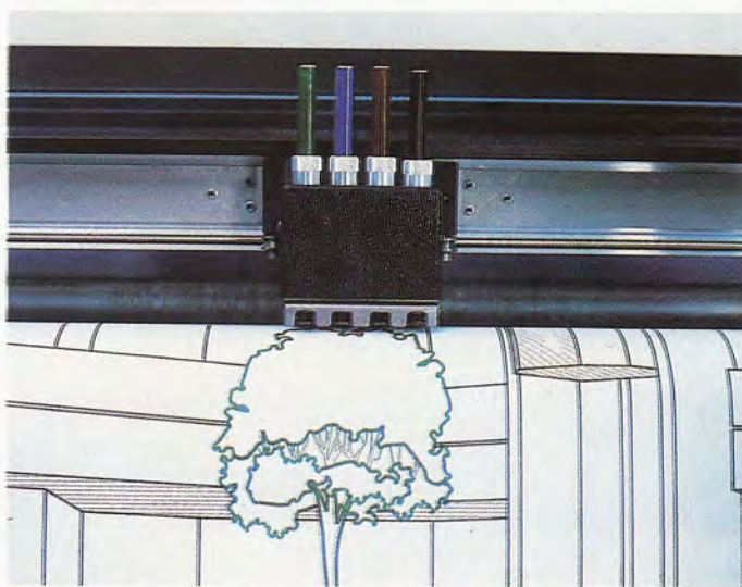
Los modelos Calcomp 965 y 970 dispones ambos de cuatro plumas que les permiten la confección de gráficos a colores.
