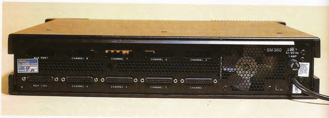
El modelo Supermux-380 permite la conexión de hasta ocho terminales en forma asíncrona. Trabaja en modo full-dúplex, y las velocidades pueden seleccionarse individualmente para cada canal.
