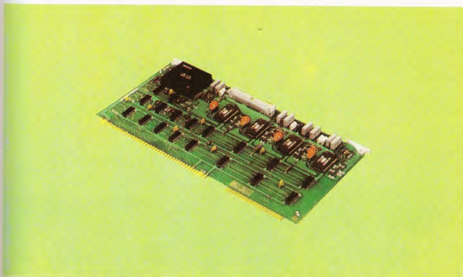
Los ordenadores en los que se implantan las tarjetas industriales gestionan sus entradas y salidas de muy diversas formas. Las Bur Brown están diseñadas de forma que los diversos canales ocupan posiciones contiguas de memoria RAM.
