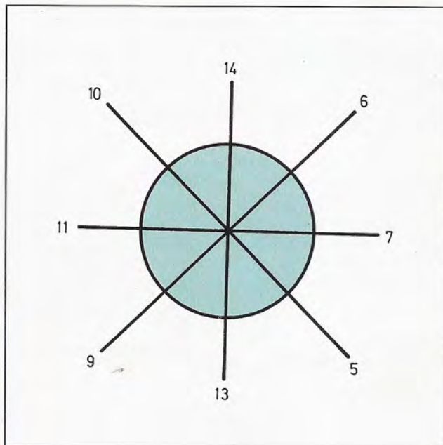
Valores devueltos por la función STICK del Basic de los ordenadores Atari, de acuerdo a los posibles movimientos de la palanca de control del joystick.
