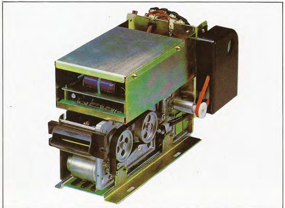
El modelo 3S4YR-PAW2 es el resultado de combinar un lector de tarjetas magnéticas con una impresora. Los datos contenidos en la tarjeta pueden ser leídos y escritos; además del equipo puede escribir sobre tarjetas magnéticas de papel.
