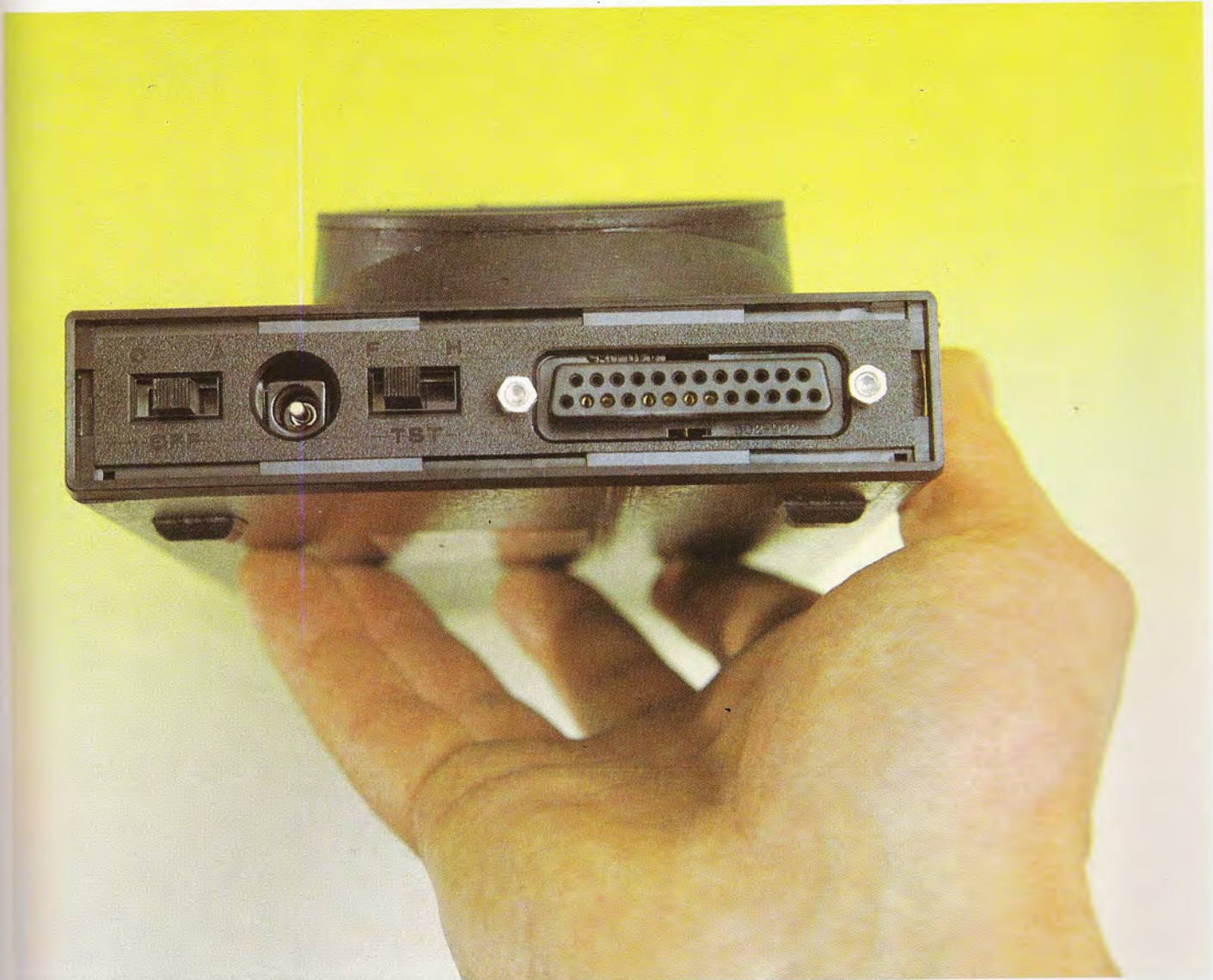
El interface para comunicación con el ordenador es de tipo serie RS/232.
