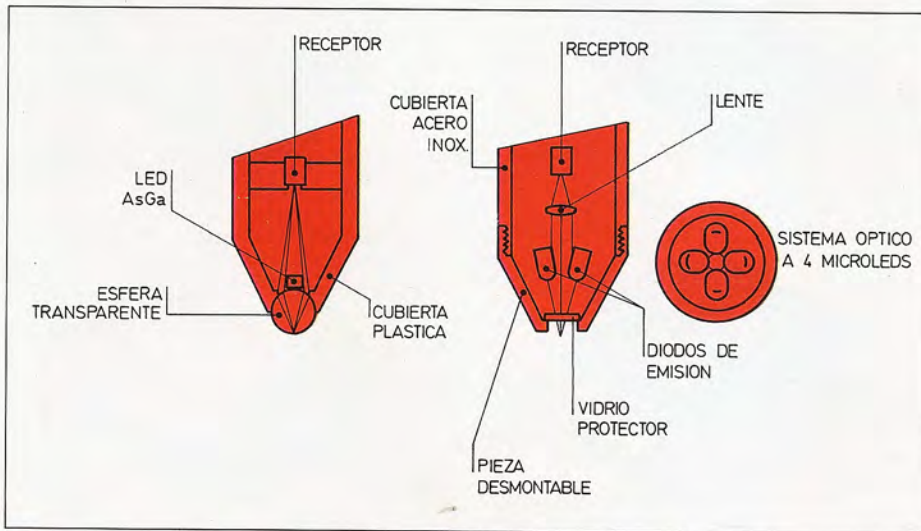
En los lectores estáticos la fuente de luz va instalada en una especie de lápiz cuya punta será esférica o plana, según el sistema óptico utilizado.
