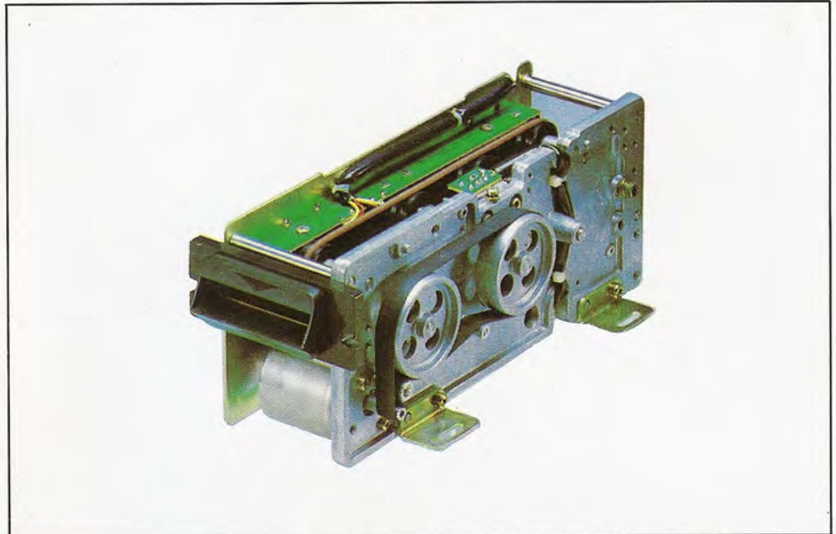
El lector de tarjetas magnéticas modelo 3S4YR-MA es de tipo motorizado y lee automáticamente los datos almacenados en la banda magnética cuando la tarjeta se coloca en la ranura correspondiente. Entre sus múltiples aplicaciones cabe destacar la de los cajeros bancarios automáticos.
