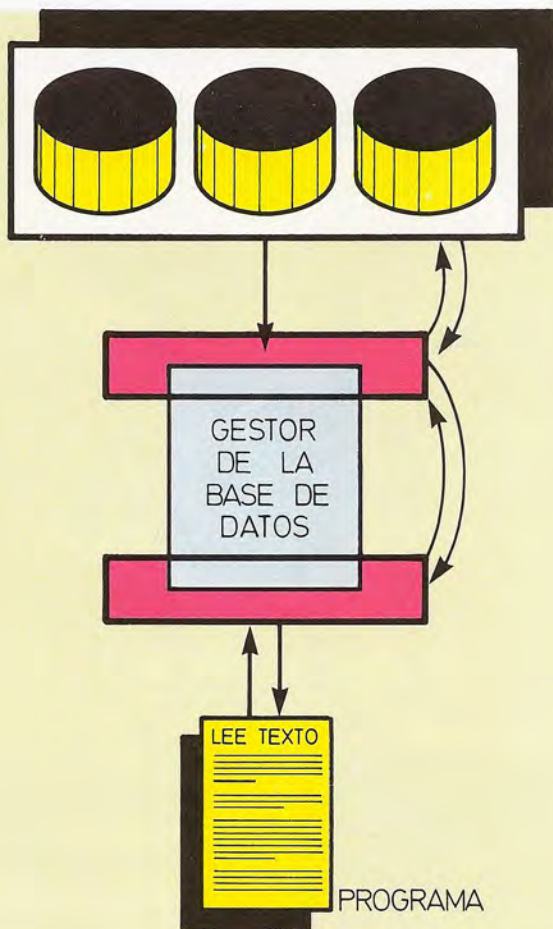
Para el sistema operativo Pick los usuarios no son más que conjuntos de ficheros. La gestión de los mismos se realiza como si se tratase de una «base de datos».
