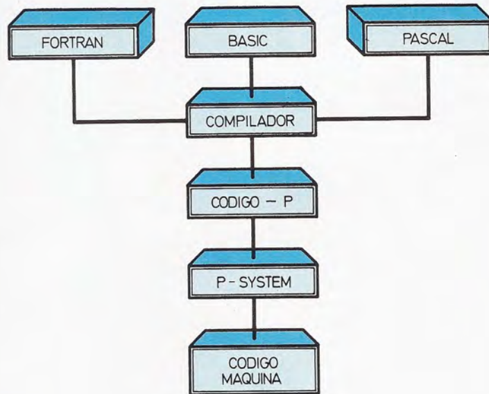
Los compiladores del UCSD p-System producen un único código, el código-p que puede traducirse a código máquina.
