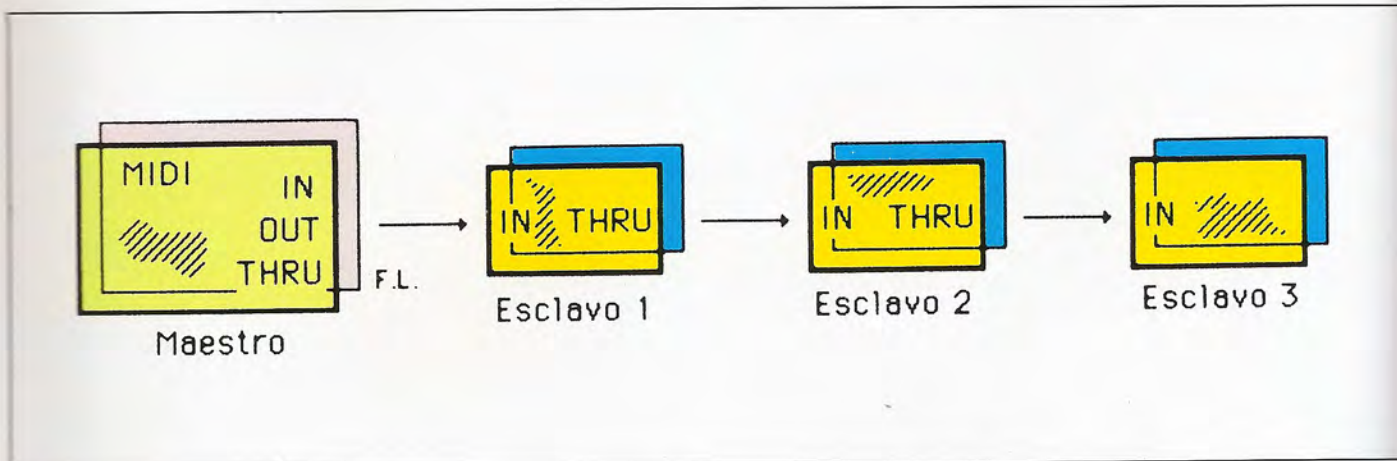
■ Sistema MIDI conectado en serie. La salida del instrumento se conecta a la entrada del primer esclavo, y la salida THRU de éste a la entrada del esclavo número dos. Esta última conexión, se repite para los restantes, hasta un máximo de tres o cuatro.
