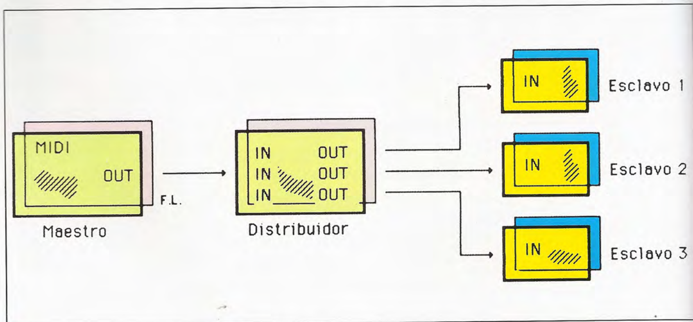
■ Conexión en estrella de un sistema MIDI. La salida del maestro se lleva a un distribuidor al que se conectan todos los esclavos. El número máximo de estos está limitado únicamente por el número de salidas del distribuidor.
