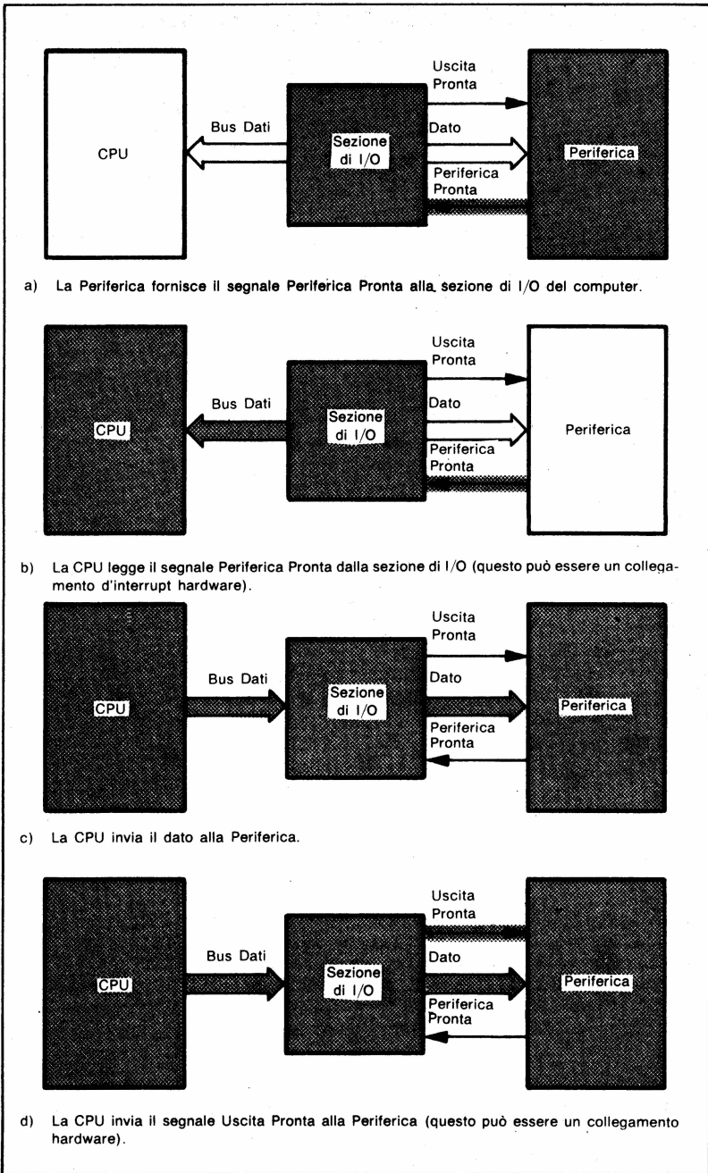
Figura 11-6. Un Handshake di Uscita
