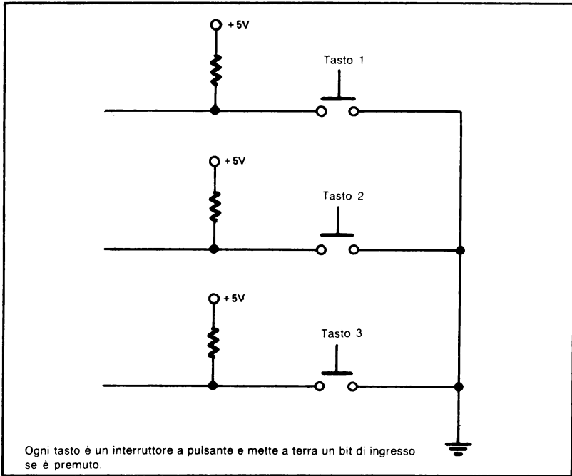
Figura 11-20. Una Piccola Tastiera
