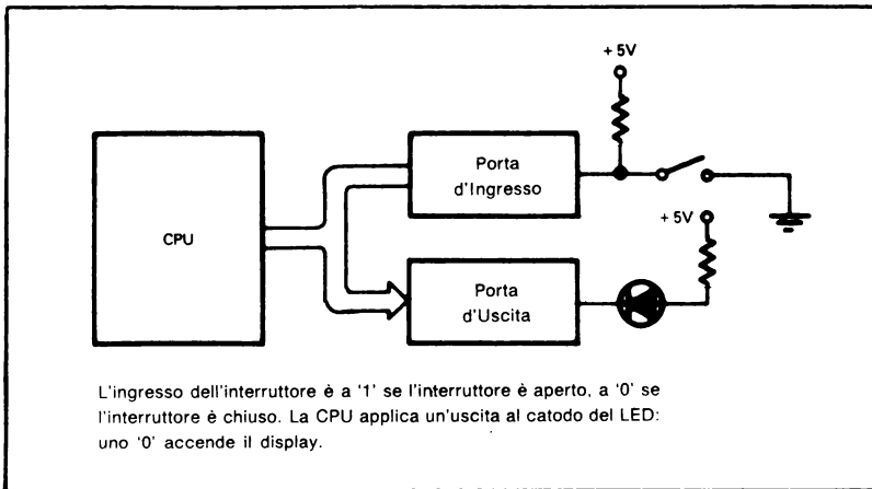
Figura 13-2. Il sistema Interruttore-Display
