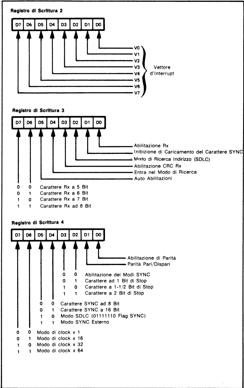
Figura 11-33. Controllo del SIO o Registri di Scrittura (continua)
