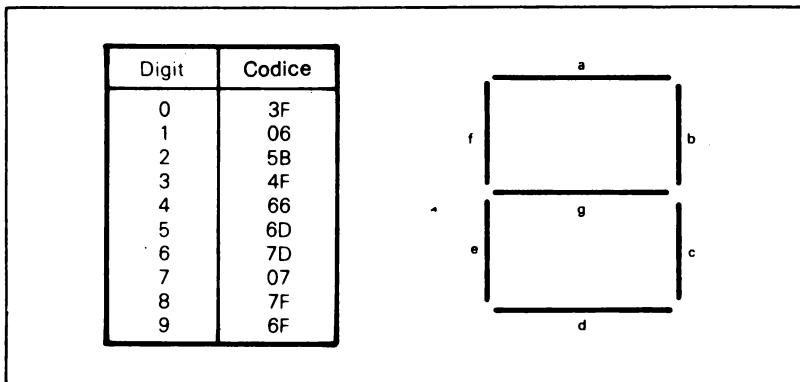
Figura 7-1 Combinazione dei sette segmenti
