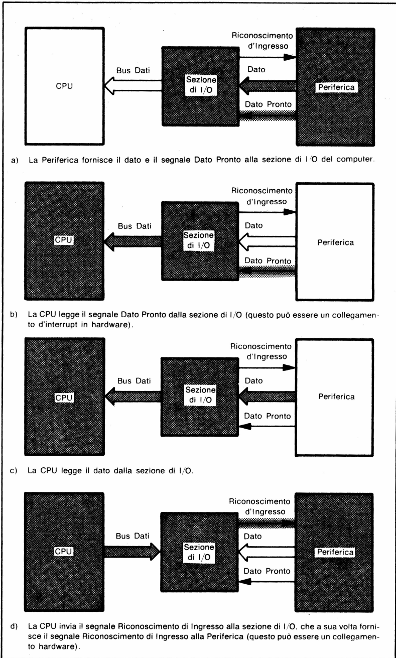
Figura 11-5. Un Handshake di Ingresso.
