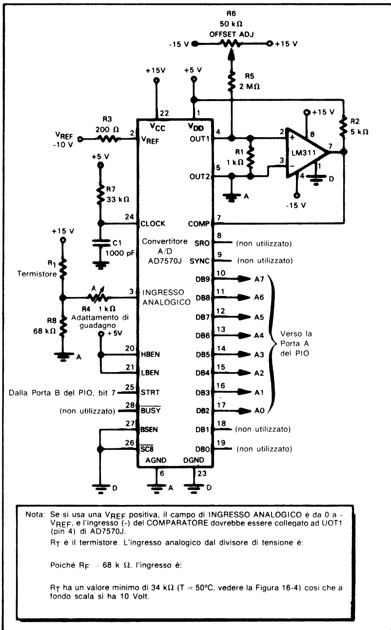
Figura 16-3. Hardware Relativo al Termometro Digitale
