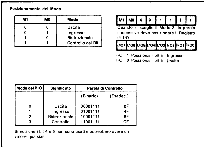
Figura 11-9. Controllo del Modo per lo Z80 PIO
