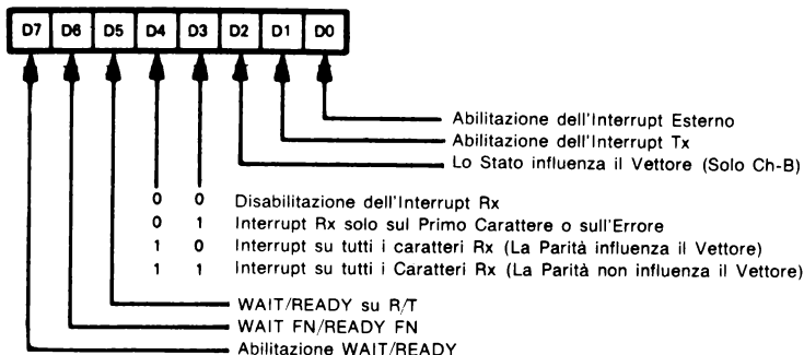
Figura 11-33. Controllo del SIO o Registri di Scrittura
