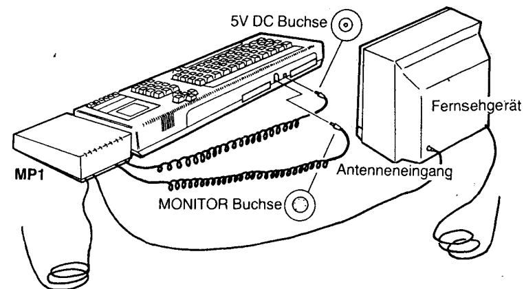
Bild 2: Anschluß von MP1, Computer und Farbfernseher.
