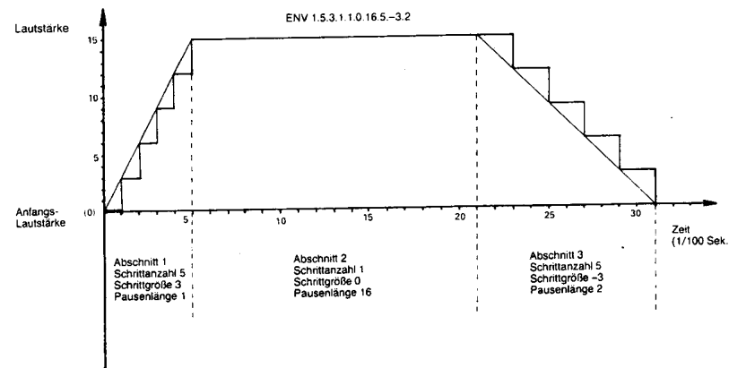
Bild 3: Beispiel für die Lautstärken-Hüllkurve
