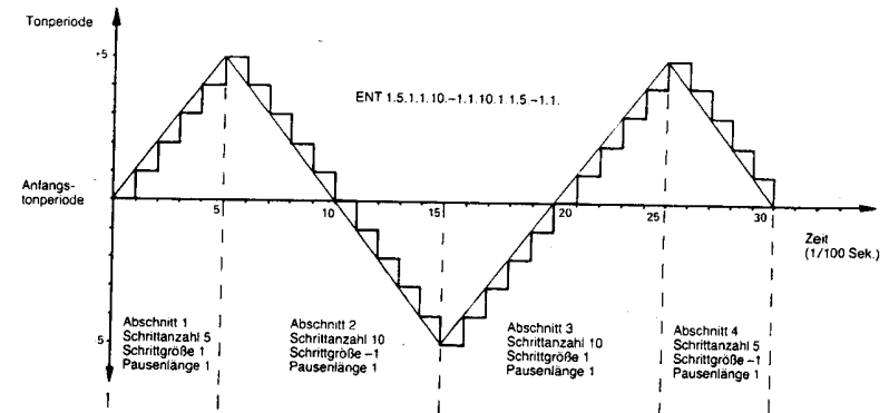
Bild 4: Kennlinie einer Ton-Hüllkurve
