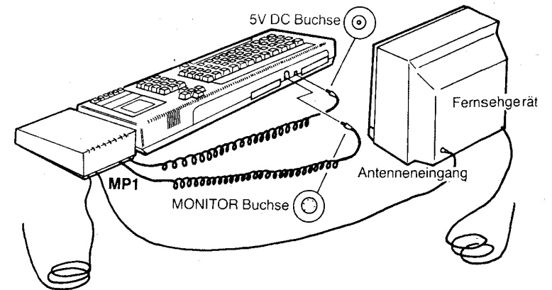
Bild 2: Das MP1 – Modulator und Stromversorgung
