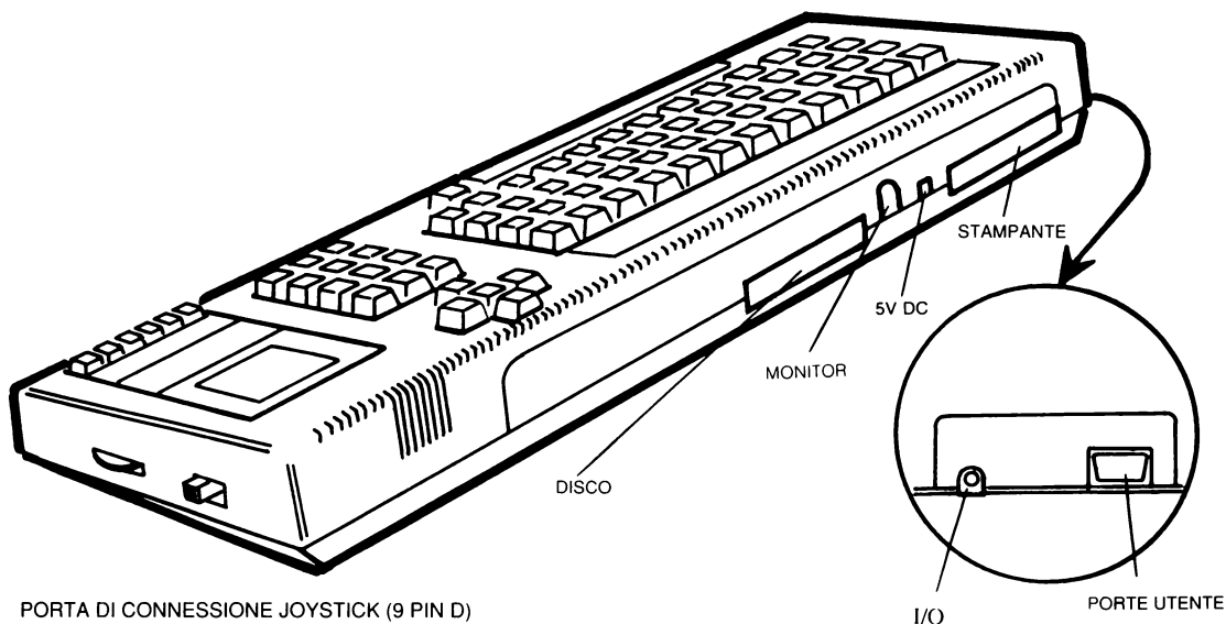
PORTA DI CONNESSIONE JOYSTICK (9 PIN D) VISTO DAL RETRO
