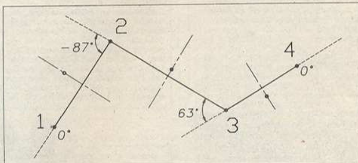
Slika 1: U tačkama 1 i 4 uglovi iznose 0 stepeni, u tački 2-87 stepeni, a u tački 363 stepena. Ako je zbir uglova negativan, on predstavlja odmicanje od simetrale u jednu stranu, a ako je pozitivan, u drugu. Generisane su tri nove tačke, što znači da ih sada ukupno ima 7 (2 \times 4 - 1 = 7) .
