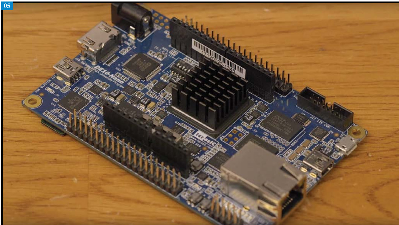
05. La DE10-Nano, la placa que sirve como base de MiSTer es en realidad una mezcla de procesador por hardware (un ARM A9 dual core), conectores (incluido para Arduino), memoria DDR3, conectores GPIO o la FPGA de Altera, Cyclone V. Imagen: V2.fi.
