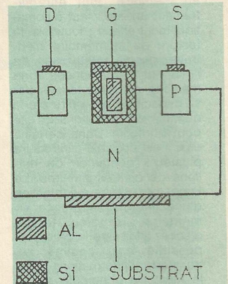
Une EPROM (Fig. 3)
