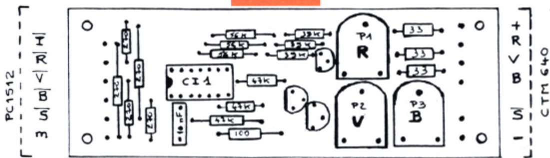
Côté composants
