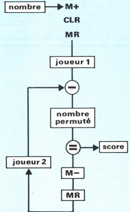
figure 2 : organigramme d'un tour de « Mutations ».
