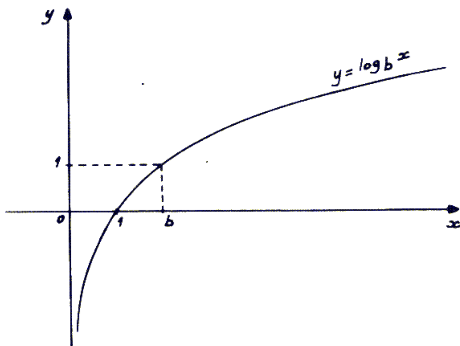
Courbe représentative de la fonction logarithme
