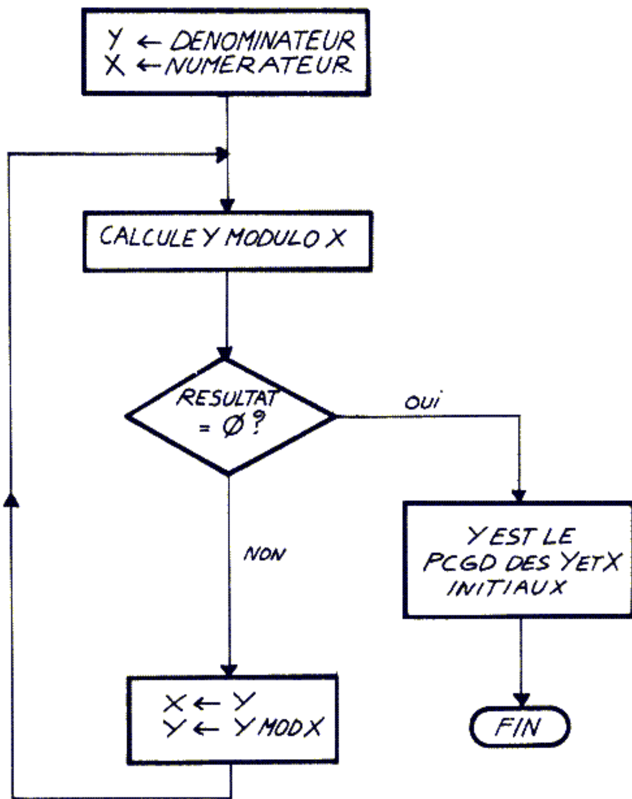
Figure 1 Algorithme de simplification de fraction dressé par Arnaud Peruta. Y et X correspondent aux registres de la pile opérationnelle.
