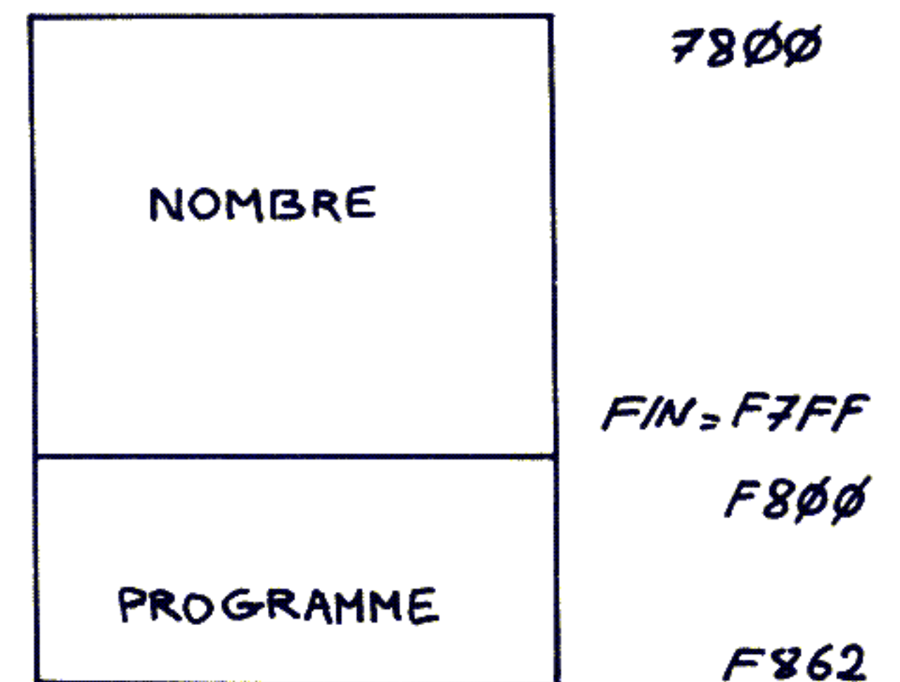
Occupation de l'espace mémoire
