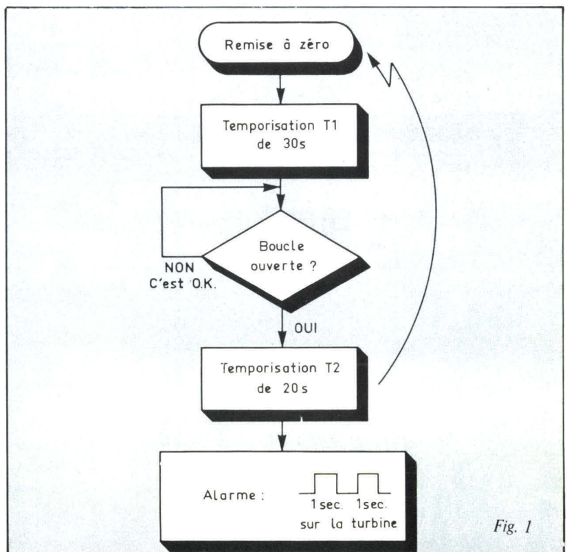
Fig. 1. - Organigramme simplifié de l'alarme.
