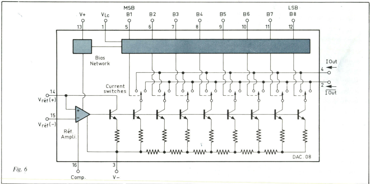
Fig. 6. - Constitution du DAC-08 : convertisseur digital-analogique de 8 bits. Les résistances du réseau R/2 R ont été ajustées au laser.
