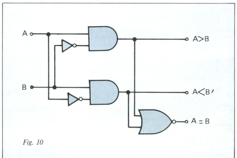
Fig. 10. - Comparateur : La fonction A = B est définie par \overline{A \oplus B} . La fonction A > B est définie par A \bar{B} . La fonction A < B est définie par \bar{A} B .
