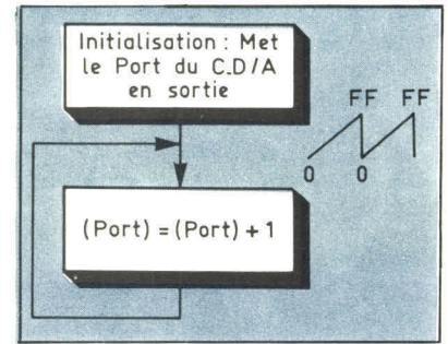
Fig. 8. - Organigramme de réalisation d'une dent de scie. Le contenu du mot mémoire présent dans le port de sortie est incrémenté.
