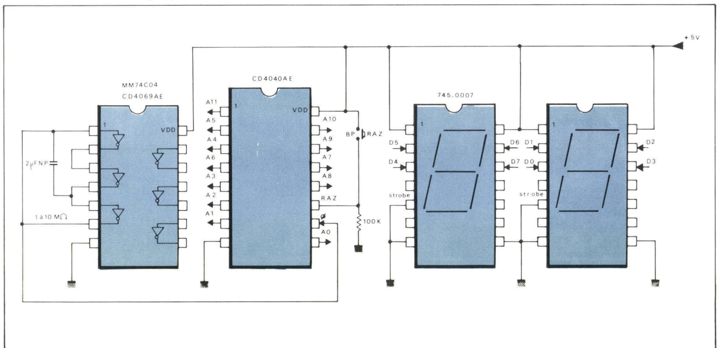
Fig. 2. - Affichage des données dans le cas d'une mémoire à mots de 12 bits codés en octal. Remarquez que toutes les entrées « D » des afficheurs sont reliées à la masse puisque la base de numération est 8.
