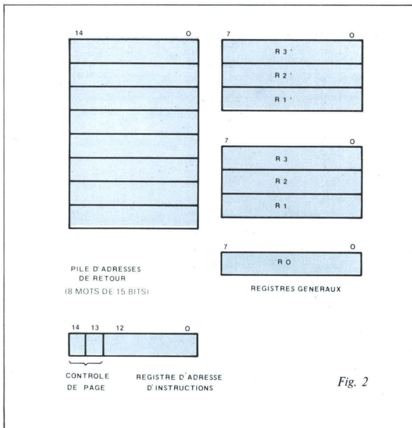
Fig. 2. - Le « 2650 » possède 7 registres généraux, une pile de 8 doubles registres et un mot d'état.
