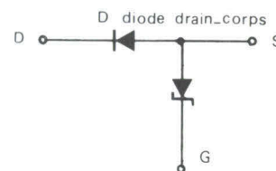
Fig. 8. - Circuit équivalent à l'état OFF ( V_{GS} = 0 ).
