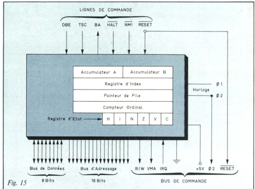
Fig. 15. - Structure interne d'un microprocesseur standard de 8 bits : le 6800.
