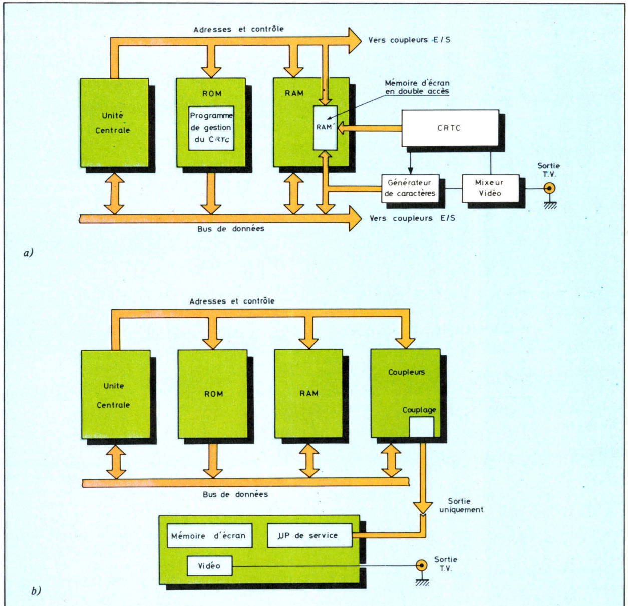
Fig. 1. - Deux méthodes de visualisation de texte : a - par vidéo RAM ou V.RAM b - à processeur spécialisé et mémoire d'écran indépendante de l'unité centrale.
