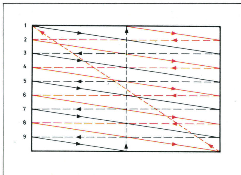
Fig. 3. - Principe du balayage entrelacé, pour un nombre impair de lignes (625). Les retours de spot en extinction sont représentés en pointillés.
