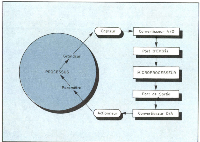
Fig. 1. - Boucle représentative de toute application. Lors du contrôle d'un processus, il faut mesurer un certain nombre de grandeurs physiques, prendre des décisions en fonction des valeurs et traduire ces décisions par des actions sur certains paramètres.
