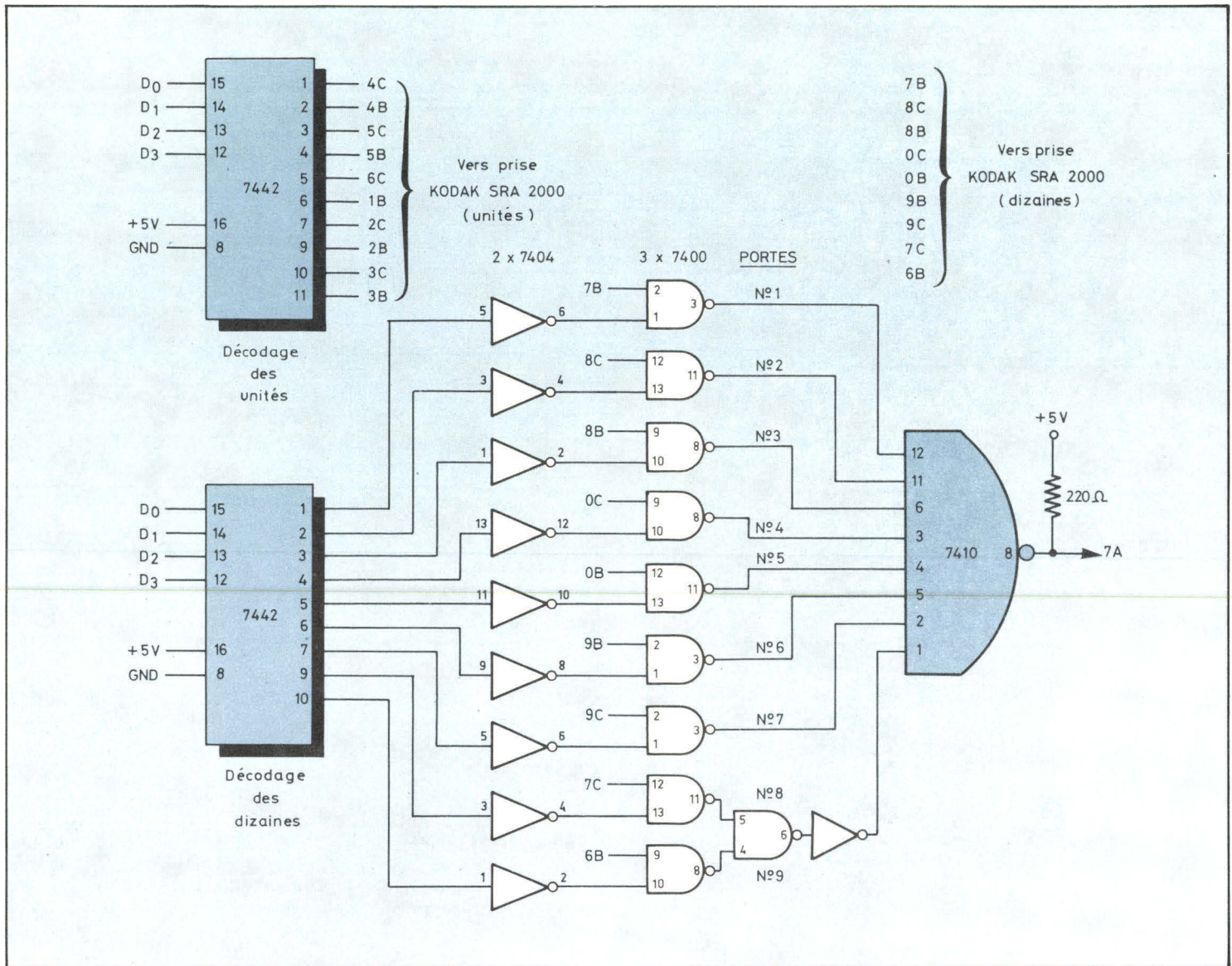
Fig. 4. - Décodage et sélection d'une diapositive. Dans l'octet mémorisé sur la carte universelle se trouve le numéro de la vue, les 4 bits de poids faible donnent après décodage (7442) le chiffre des unités et les 4 bits de poids fort celui des dizaines. Lorsque le numéro de la diapositive qui se trouve dans la fenêtre de projection coïncide avec le numéro de la diapositive sélectionnée le point 7a passe d'un niveau haut à un niveau bas et le magasin s'arrête.
