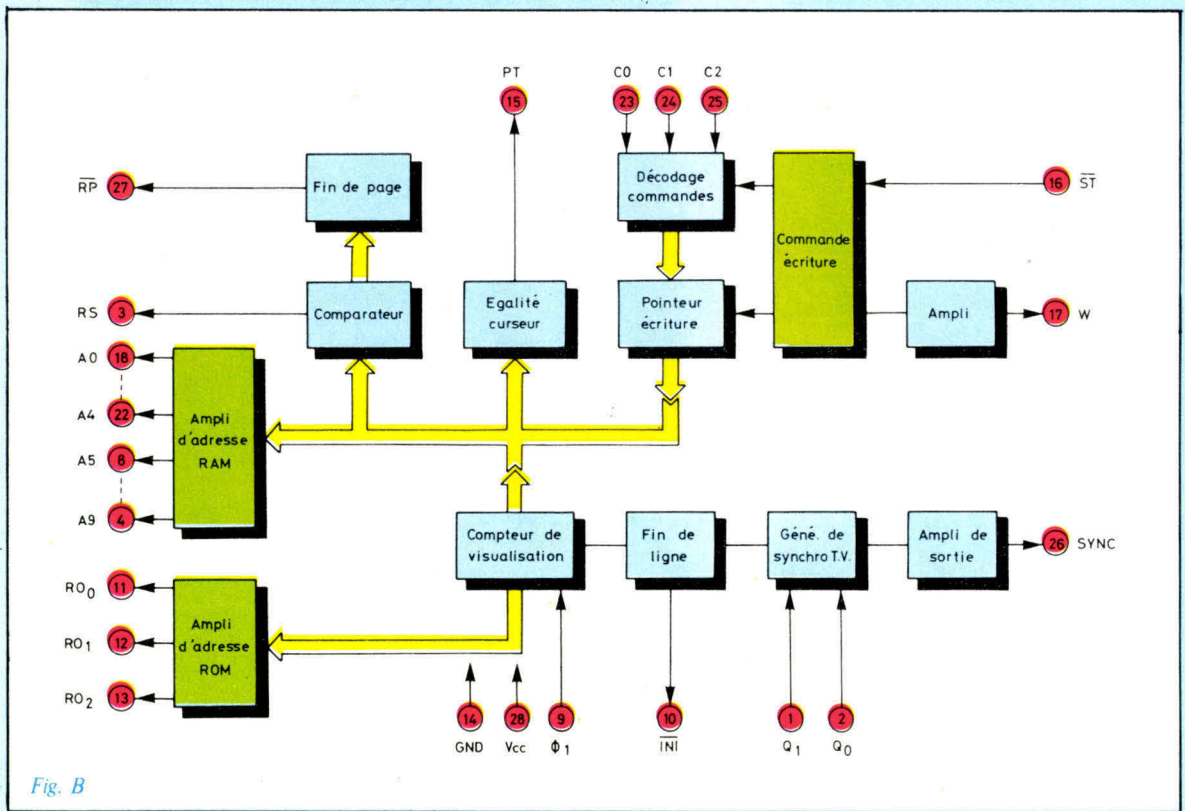
Fig. B. - Schéma synoptique du contrôleur de CRT SFF 96.364.
