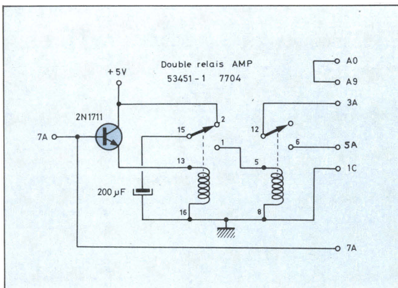
Fig. 5. - Le passage du point 7A d'un niveau bas à un niveau haut débloque le transistor et réalise l'ordre de recherche de la diapositive.
