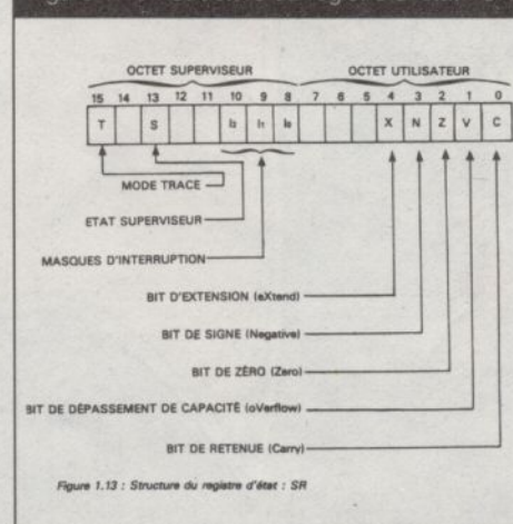
Figure 1.13 : Structure du registre d'état : SR
