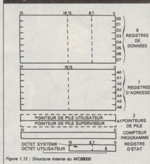
Figure 1.12 : Structure interne du MC68000
