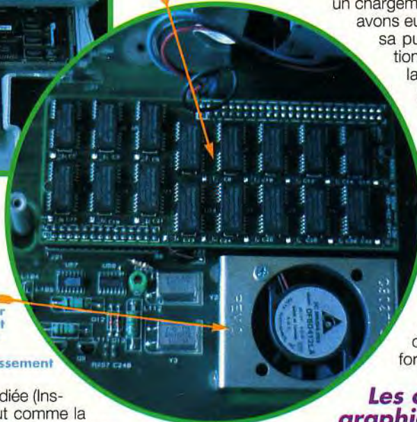
La carte mémoire n'utilise pas de composants spécifiques mais l'emploi de barrettes SIMM est préférable.
