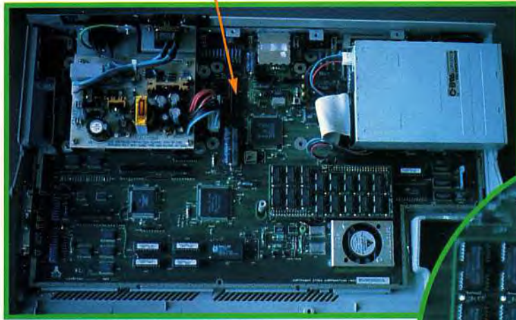
L'organisation de la carte du Falcon 030 s'apparente à celle des STF/E.
