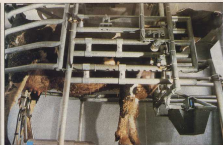
La traite en self-service, c'est possible avec le robot à quatre bras du Cemagref d'Antony.
