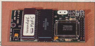
Le modem Amazone version coffret de PNB. La platine piggy back du contrôleur MNP 5 de PNB.
