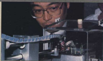
Des ressorts en alliage à mémoire de forme pour cueillir de grêles plantules.
