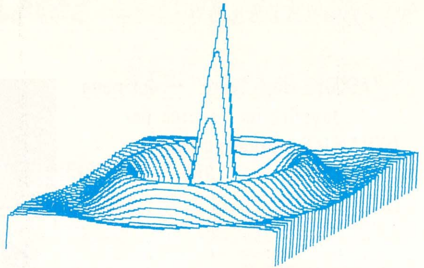
Sogenanntes Sombrero-Bild am Beispiel eines Co-tangens
