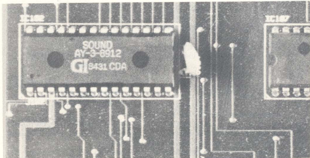
Der Tongenerator-Baustein AY-3-8912 von GI ermöglicht dreistimmige Tonerzeugung. Der Ton aller 3 Kanäle wird gleichmäßig gemischt und über den eingebauten Lautsprecher ausgegeben. Die Anschlußmöglichkeit an eine Stereo-Anlage ermöglicht optimale Klangeffekte, wobei Kanal C gleichmäßig auf die anderen beiden (A + B) verteilt wird.
