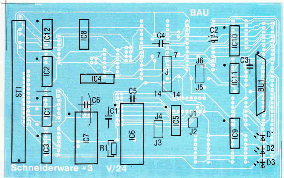
Bestückungsplan
