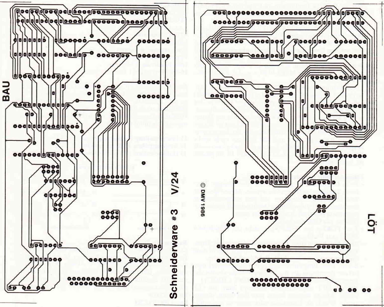
Repro 1+2: Platinenlayout
