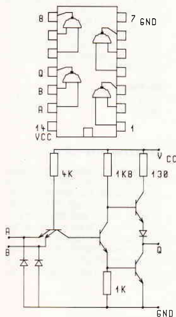
Bild 1: Innenschaltung 7400
