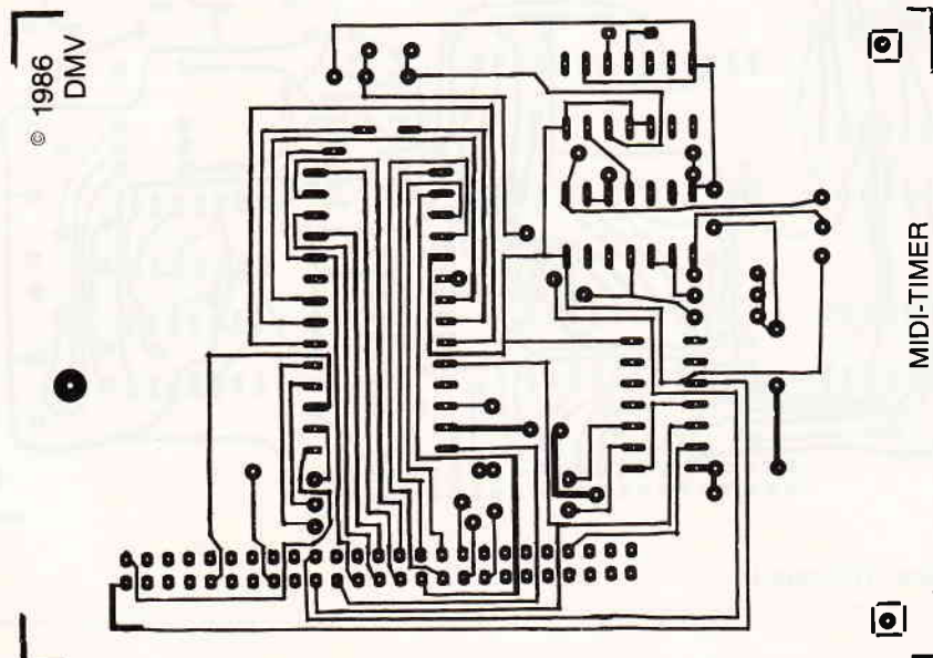
Bild 10: Layout des Timers (Lötseite)
