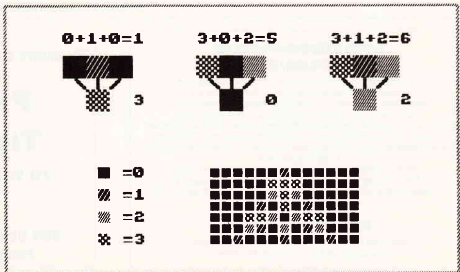
Bild 1: So arbeitet der eindimensionale Zellautomat
