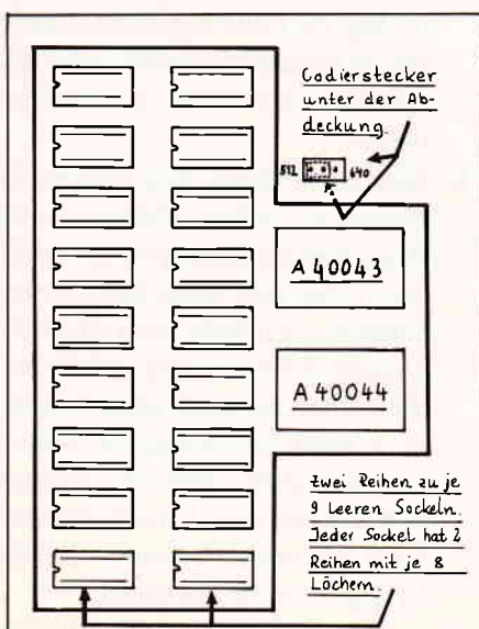
Abb. 3: Ansicht der leeren IC-Sockel
