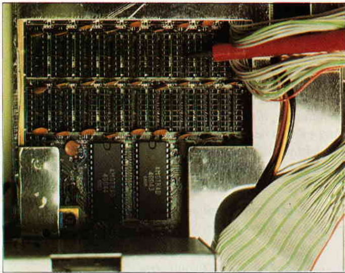
Der RAM-Speicher des PC 1512 kann auf der Hauptplatine bis 640 KB aufgerüstet werden. Wie dieses selbst realisiert werden kann, zeigt Ihnen unser aktueller Bericht.
