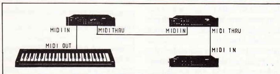
Abbildung 4: Expander - Einsatz
