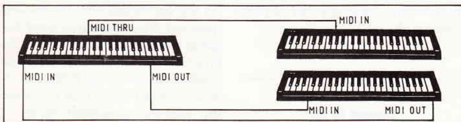
Abbildung 3: MIDI THRU im MIDI-Verbund
