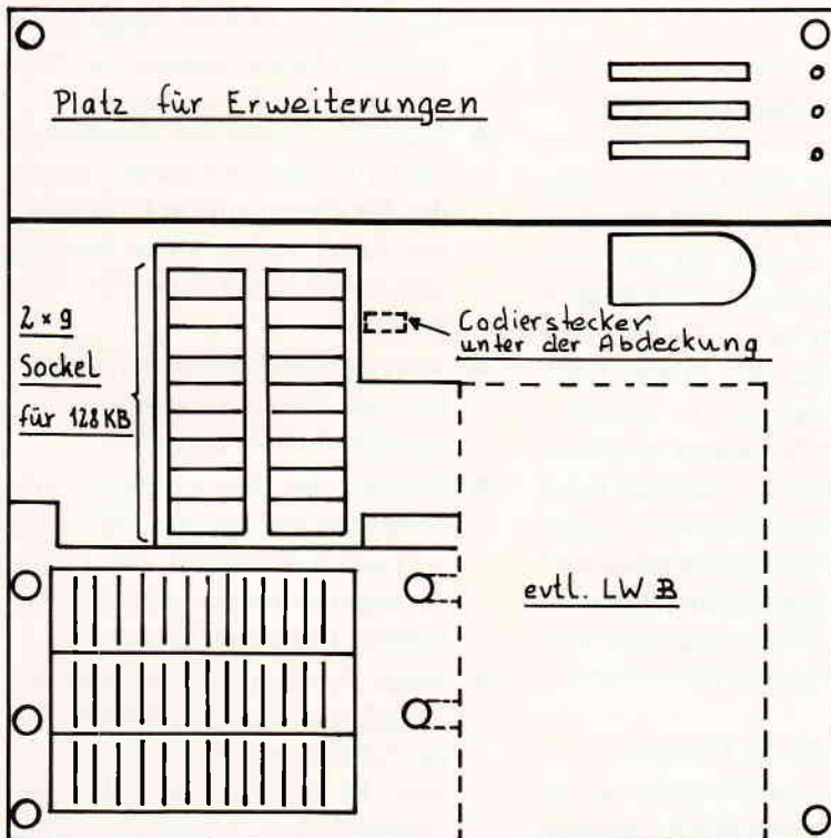
Abb.2: Ansicht des CPU-Innenraums
