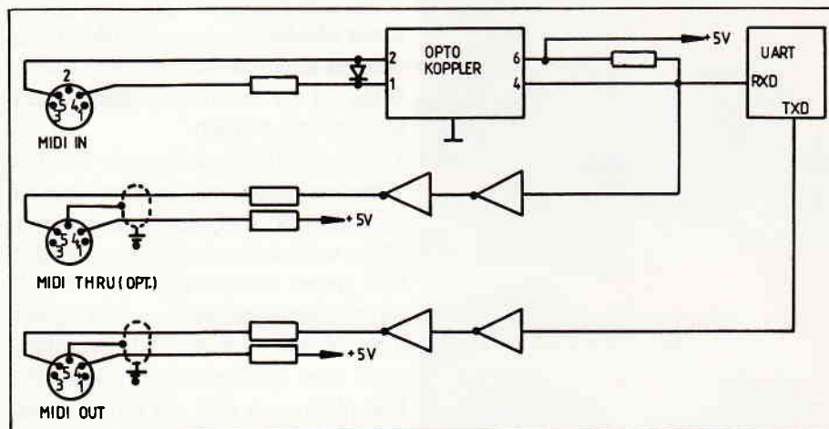
Abbildung 1: Die MIDI-Hardware
