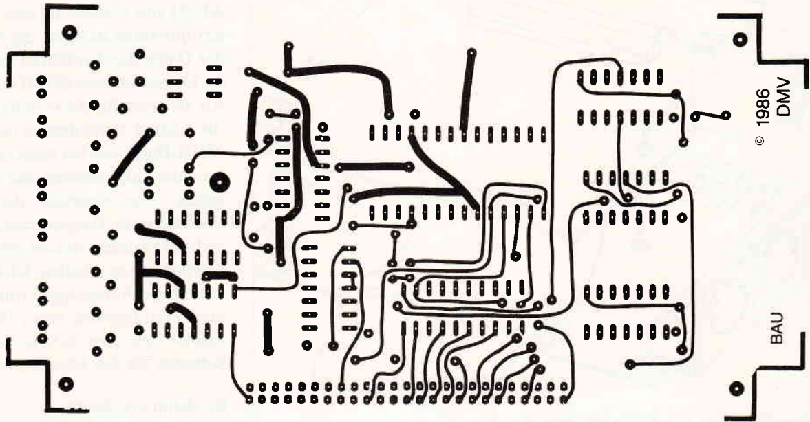
Bild 9: Layout des Interfaces (Bestückungsseite)
