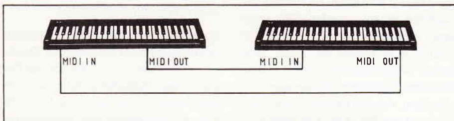
Abbildung 2: Parallelschaltung
