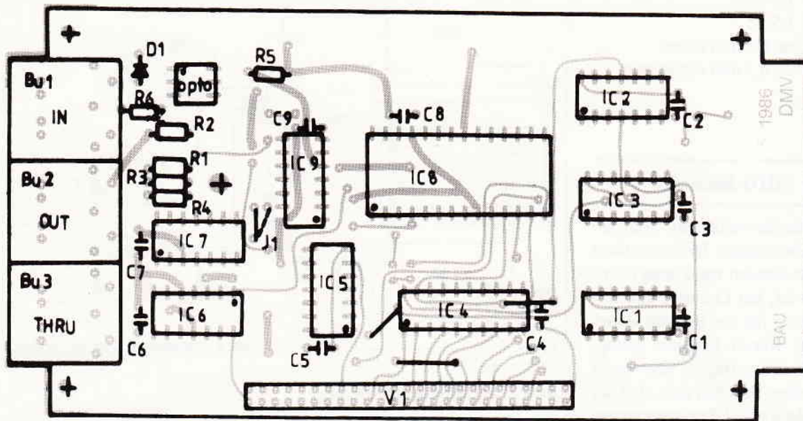
Bild 3: Bestückungsplan des Interfaces
