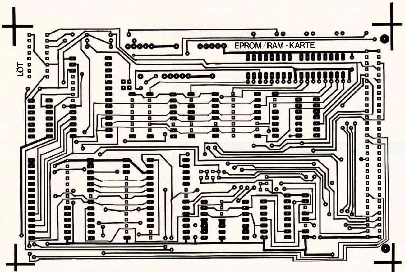
Platinenlayout Lötseite
