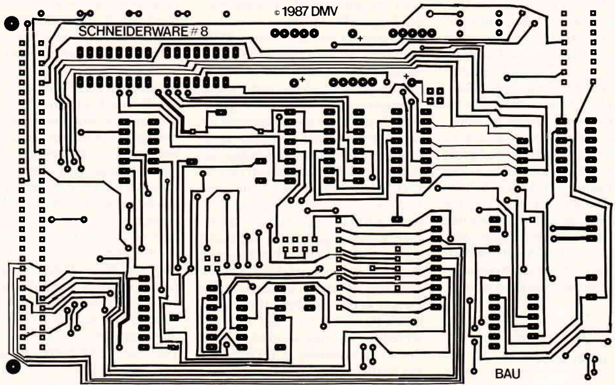
Platinenlayout Bauseite
