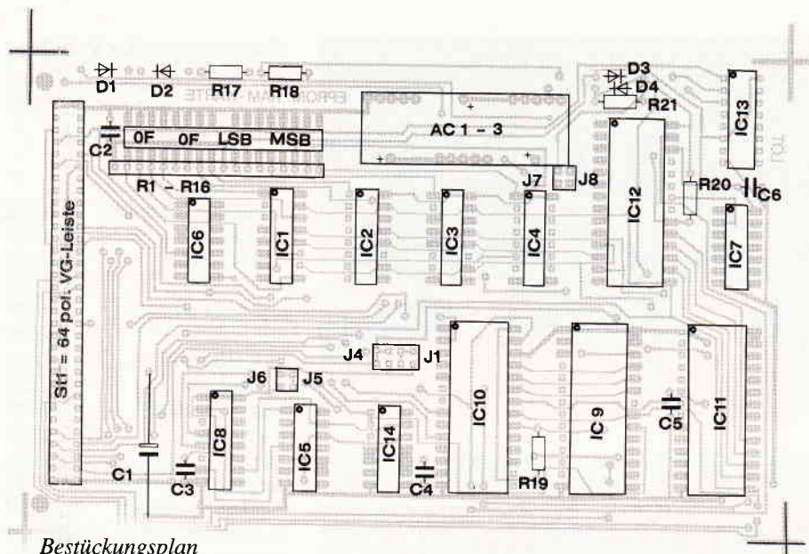
Bestückungsplan
