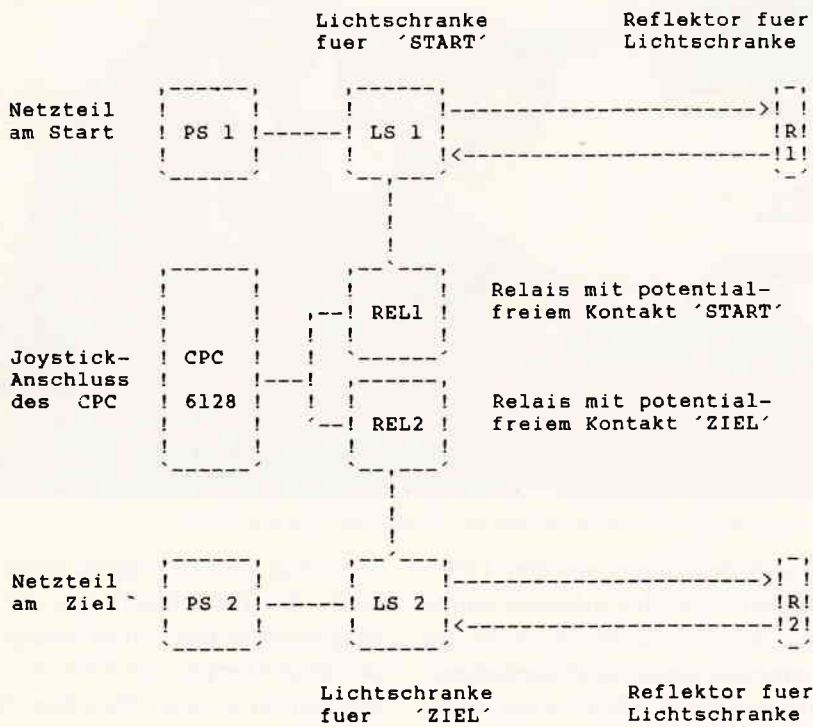
Bild 2: Hardware zum Betrieb von Race-Timer.
