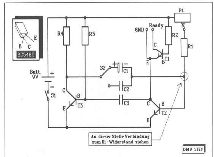
Abb. 1: Der Schaltplan zur Prozessor-Bremse
