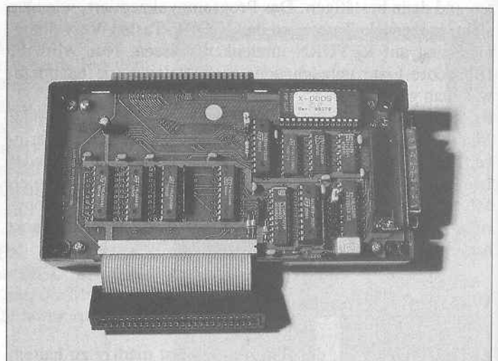
Bild 2: Der geöffnete Controller
