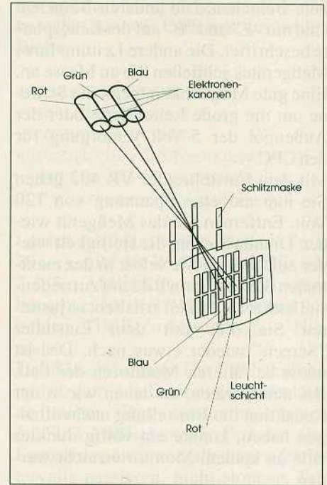
Prinzip einer In-Line-Farbbildröhre
