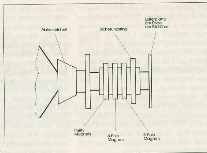
Die Anordnung der Teile auf dem Bildröhrenhals
