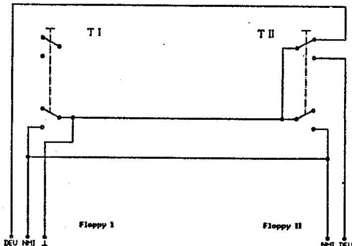
Abb. 1 Der Schaltplan
