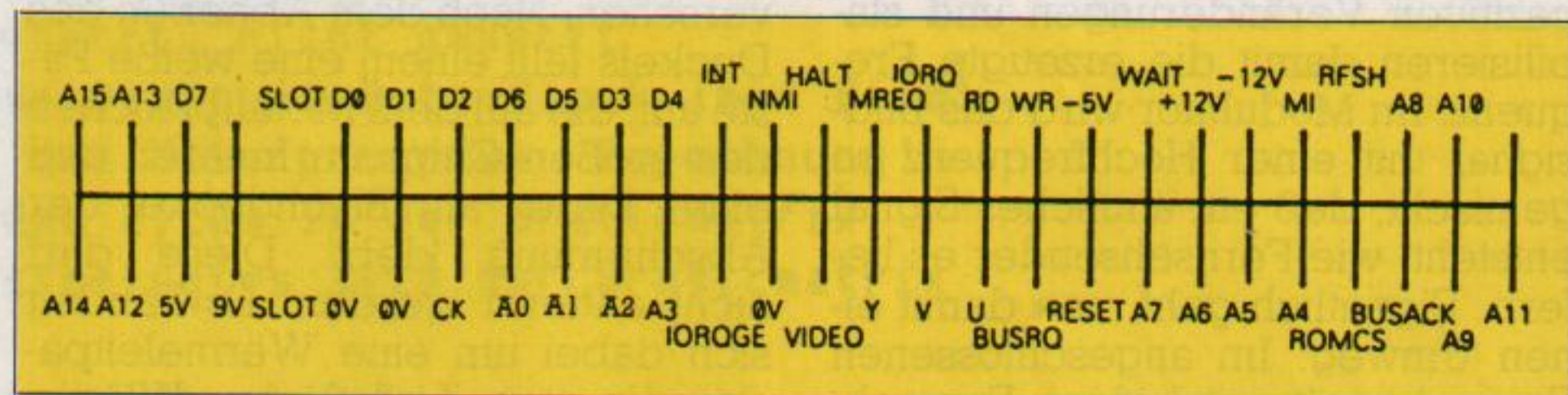
Bus-Erweiterung beim Spectrum
