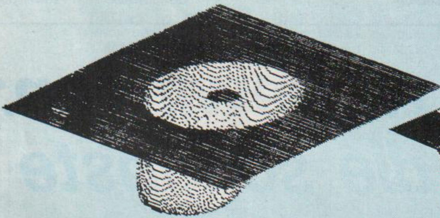
Beispiel 4: (Schnitt) wie Beispiel 3 nur ZM = -30
