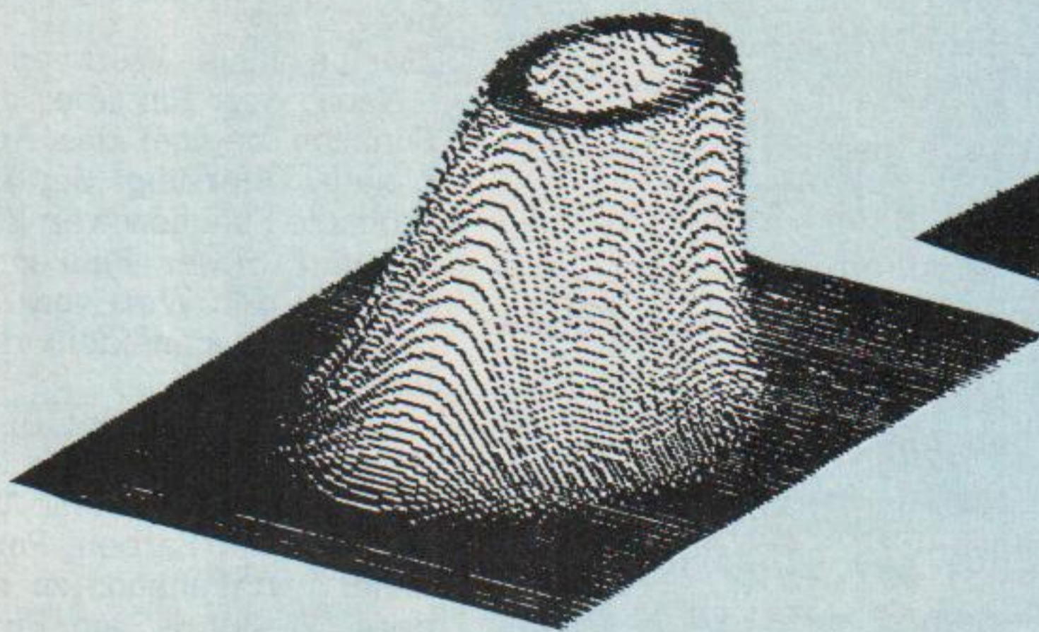
Beispiel 2: v_x = -75 , v_y = -75 , v_z = 0 , rg = 1 , sz = 13000 , ZM = 90 Funktion = (x \star x + y \star y) / 22500 \star \exp(-(x \star x + y \star y) / 450)
