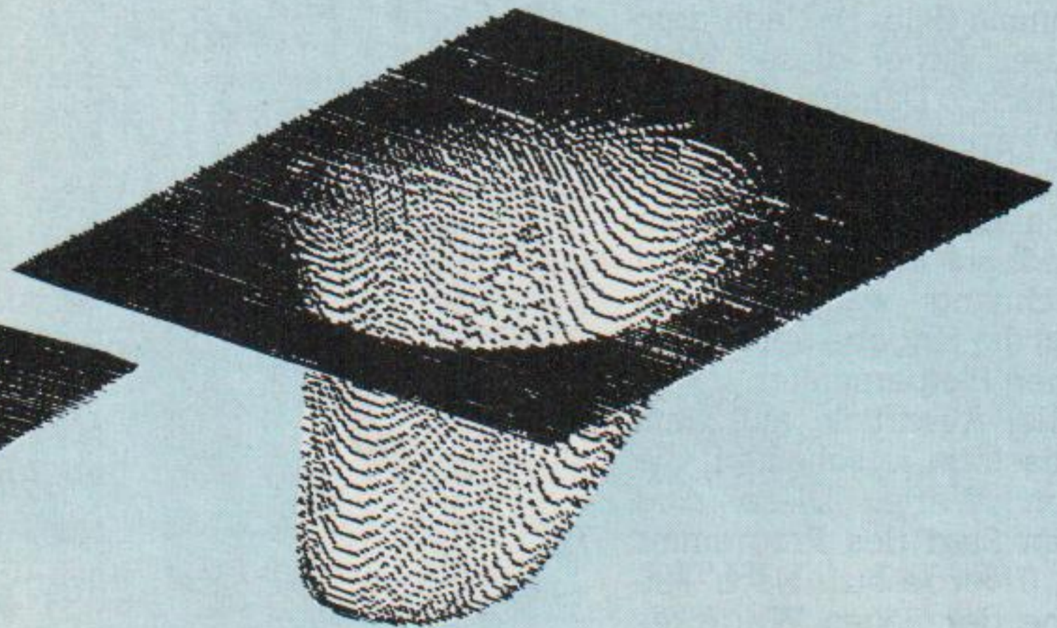
Beispiel 3: wie Beispiel 2 nur ZM = 175 und sz = -13000 , v_z = 68
