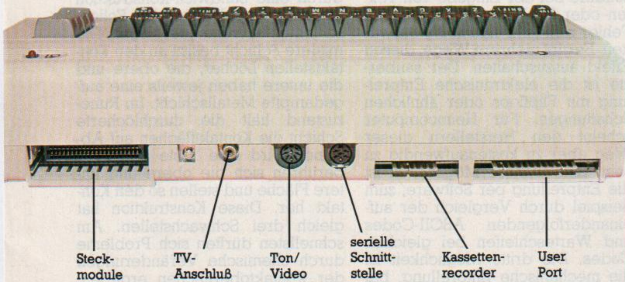
Buchsen-Beschaltung des Commodore 64, Rückseite
