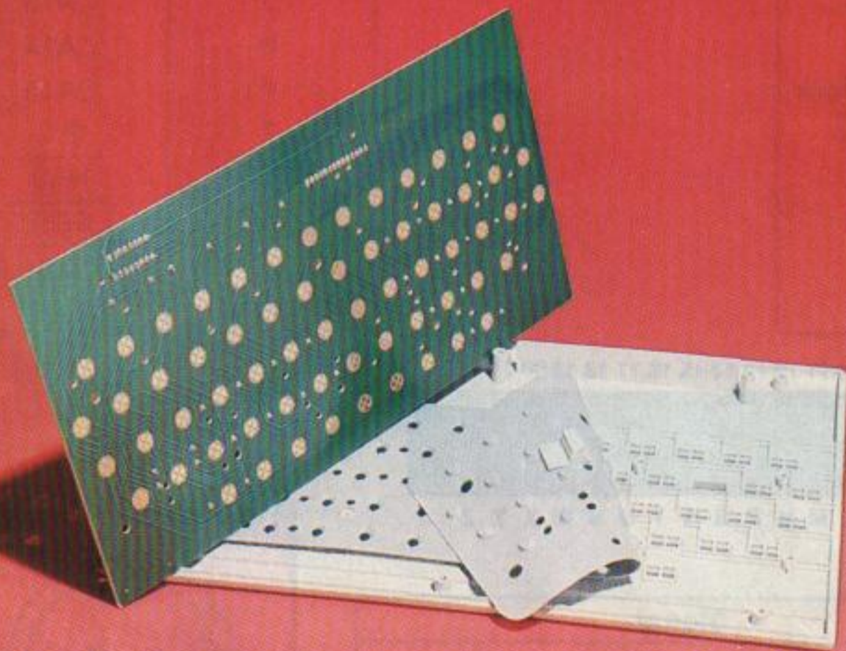
Oric-1: Tastaturplatine, Gummimatte und Hartplastiktasten
