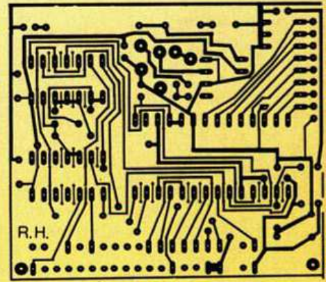
Leiterbahnseite
