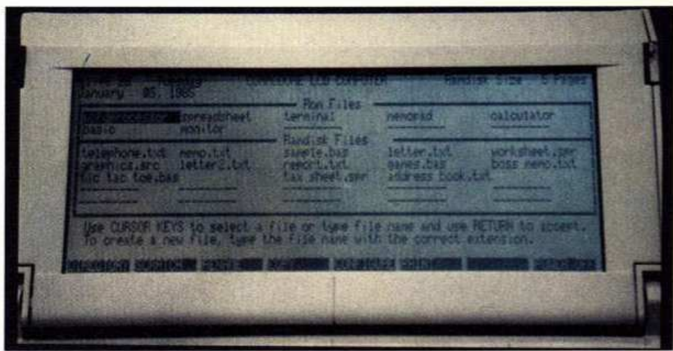
Der Tragbare von Commodore heißt Commodore LCD. Sein Display stellt 16 x 80 Zeichen in hervorragendem Kontrast dar. Rechts oben das passende batteriegespeiste 3 1/2-Zoll-Laufwerk 1571.
