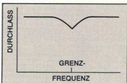
Bild 4. Bandsperre
