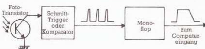
Bild 4. Einfaches Schaltungsschema des Lichtgriffels
