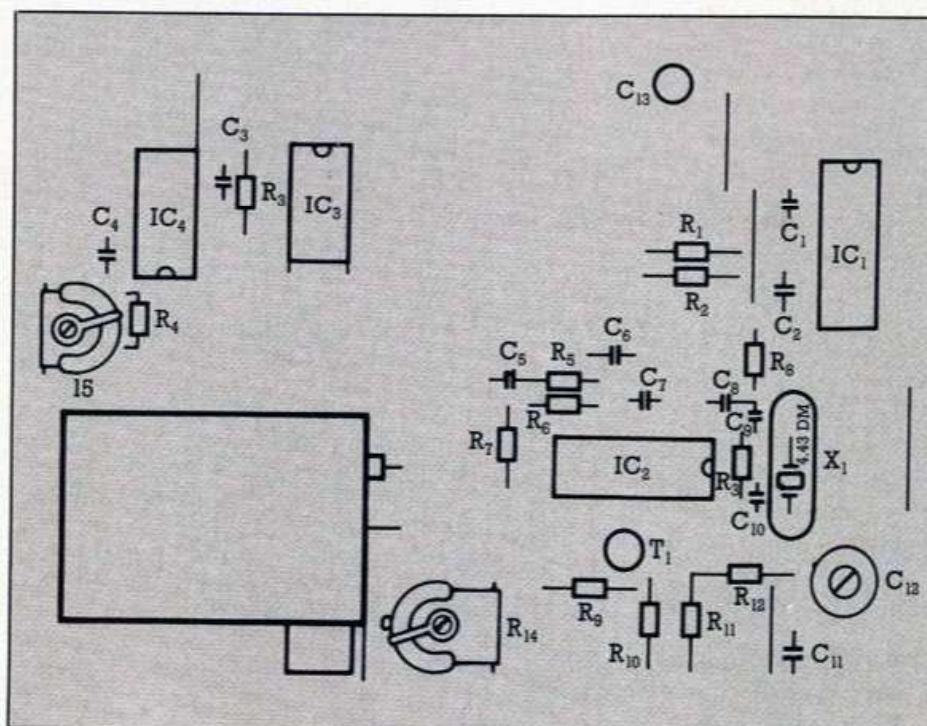
Bild 2. So gehören die Bauteile auf die Platine
