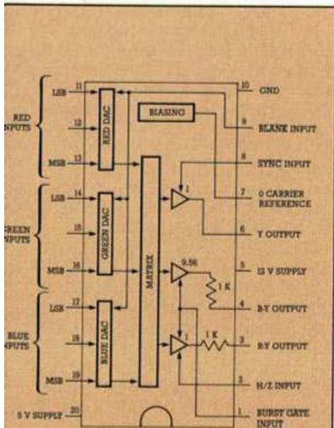
Bild 10. Digitale Eingangssignale werden von dem LM 1886 in Analogsignale gewandelt und mit verschiedenen Synchronisations-Impulsen versehen (Linear Databook, National Semiconductor)
