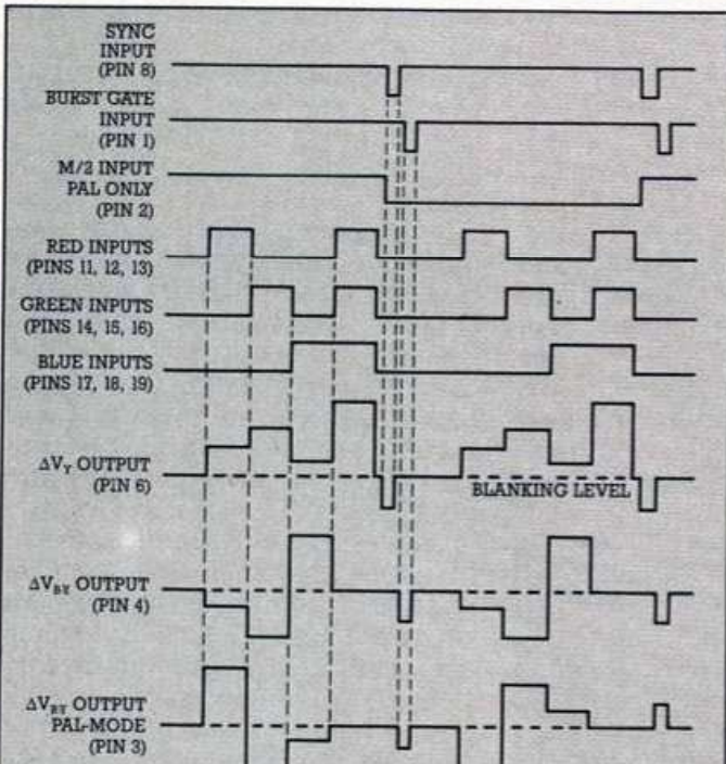
Bild 6. Das Impulsiagramm verdeutlicht die Signale des LM 1886 (Linear Databook, National Semiconductor)
