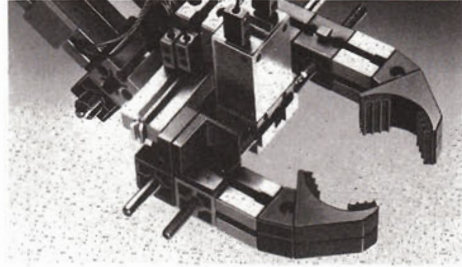
Greifhand mit symmetrischem Spindeltrieb.
