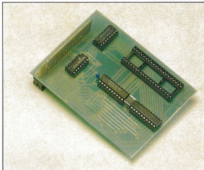
Bild 1. Musteraufbau der PIO
