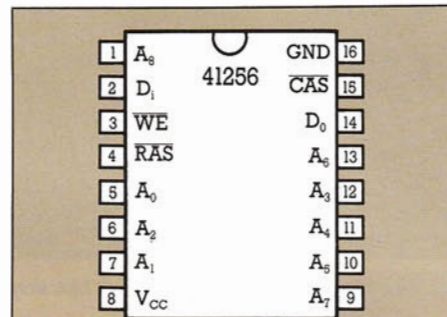
Bild 1. Anschlußbelegung eines RAM-Bausteins
