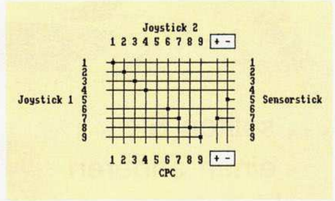
Das ist das Verdrahtungsschema für das Zusatzgehäuse
