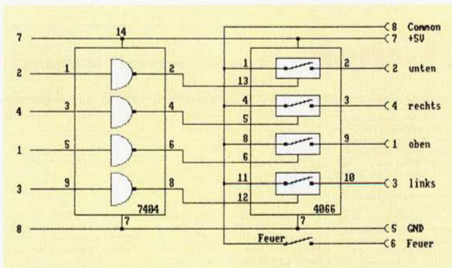
Die Zusatzschaltung besteht aus wenigen Bauteilen
