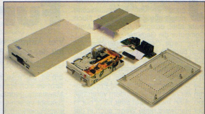
Das Diskettenlaufwerk. Die kleine Steckerplatine ist über Kabel mit dem Laufwerk verbunden.
