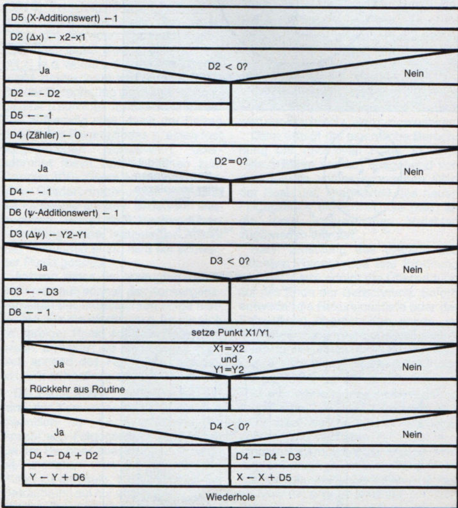
Struktogramm zur Line-Routine
