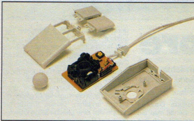
▲ Klein, aber oho! Die Maus in ihren Einzelteilen.
