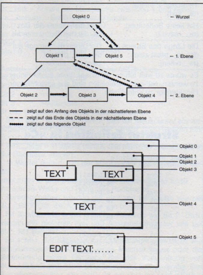
Bild 1. Objektbaum
