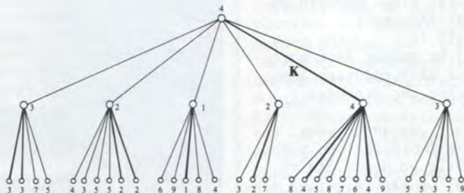
Σχήμα 2: Η μεγαλύτερη από τις ελάχιστες βαθμολογίες υπαγορεύει τη σωστή κίνηση K.
