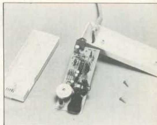
Το εσωτερικό του Voice Master Junior
