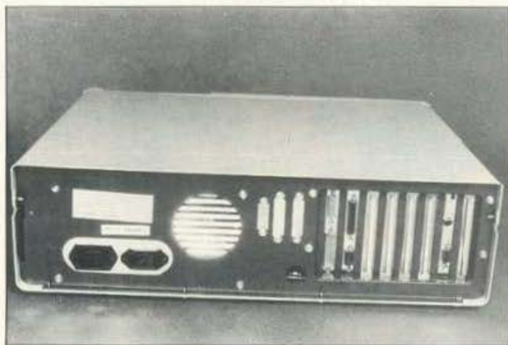
Η πίσω πλευρά του Sparrow είναι αρκετά πλούσια σε θύρες.
