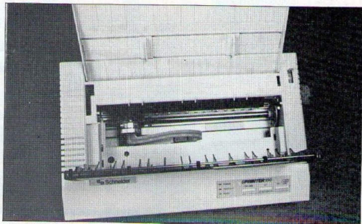
Η κεφαλή (9 pins) του εκτυπωτή. Ζεσταίνεται αρκετά.
