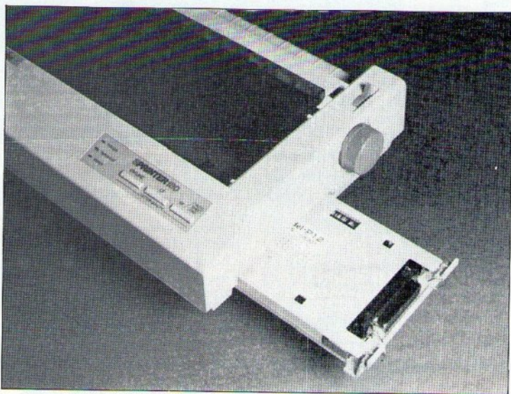
Η κάρτα που επάνω της έχει τη θύρα Centronics. Όταν την τραβήξουμε, μας αποκαλύπτει τα dip switches.
