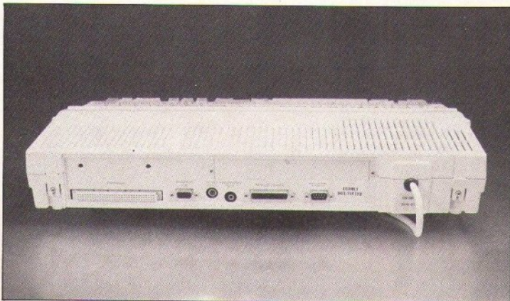
Η πίσω πλευρά του A3000, το πλούσιο σε υποδοχές, από κάθε άλλο micro. Expansion slots, υποδοχές για ακουστικά, RGB monitors, centronics, RS-232 και Econet.
