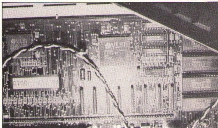
Άποψη του εσωτερικού του A3000. Πολύ πιο συμπαγής και προσαρμοσμένη κατασκευή, σε σχέση με τα παλαιότερα μοντέλα. Διακρίνεται ο ARM, το chip που εξαστολεί bits και bytes με ταχύτητα 4 Mips.
