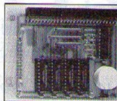
ΕΠΕΚΤΑΣΗ ΜΝΗΜΗΣ 512 KB ΜΕ REAL TIME CLOCK, ΜΠΑΤΑΡΙΑ, ΔΙΑΚΟΠΤΗ ENABLE-DISABLE, SOFTWARE RAM TEST ΠΙΑ ΤΗΝ A500
