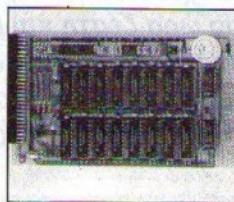
ΕΠΕΚΤΑΣΗ ΜΝΗΜΗΣ ΑΠΟ 512KB ΕΩΣ 1.8/2 MB. REAL TIME CLOCK, ΜΠΑΤΑΡΙΑ, ΔΙΑΚΟΠΤΗ ENABLE-DISABLE, SOFTWARE RAM TEST. ΠΙΑ ΤΗΝ A500.
