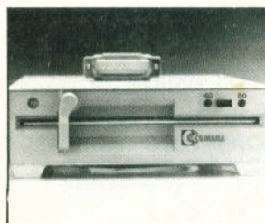
DISK DRIVES 5 1/4" 1MB/360KB/720KB/1.6MB FORMAT ΔΙΑΚΟΠΤΗ ENABLE - DISABLE » 40 - 80 TRACKS INTERNAL - EXTERNAL IBM ΣΥΜΒΑΤΑ ΓΙΑ ΤΗΝ A500 - 2000
