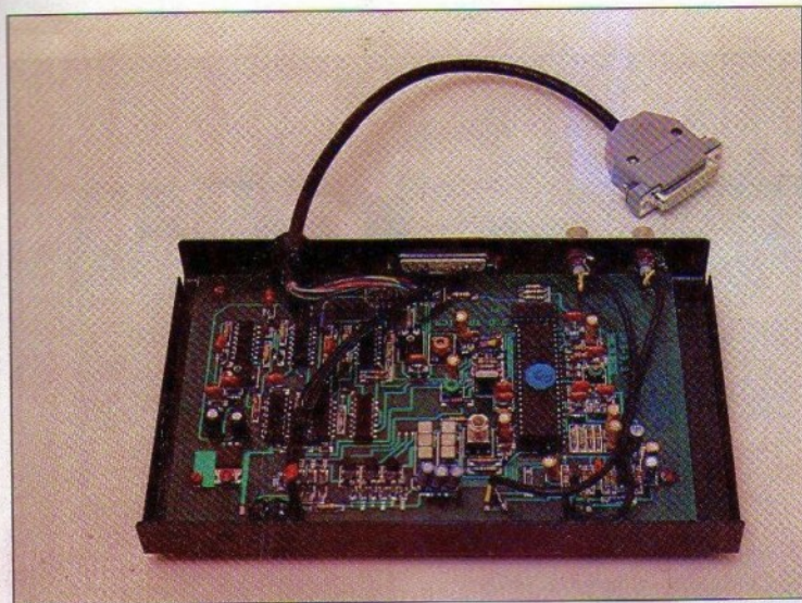
Το εσωτερικό του "μικρού" Genlock.
